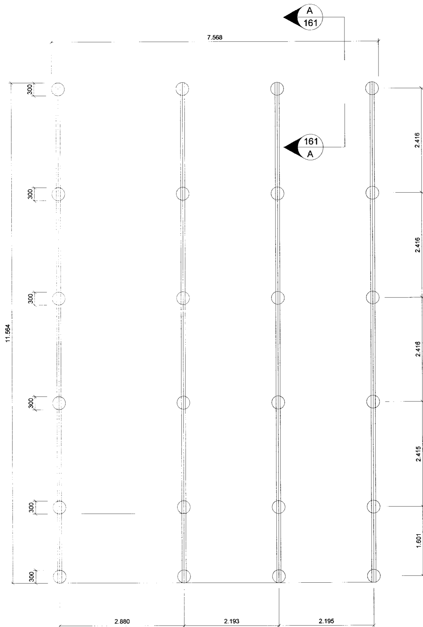
Grunnmynd, súluplan mkv. 1:50
