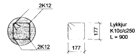
B Sneiðing 161 1:20
