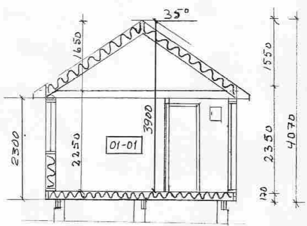
A M 1:50 Sneiðing A
