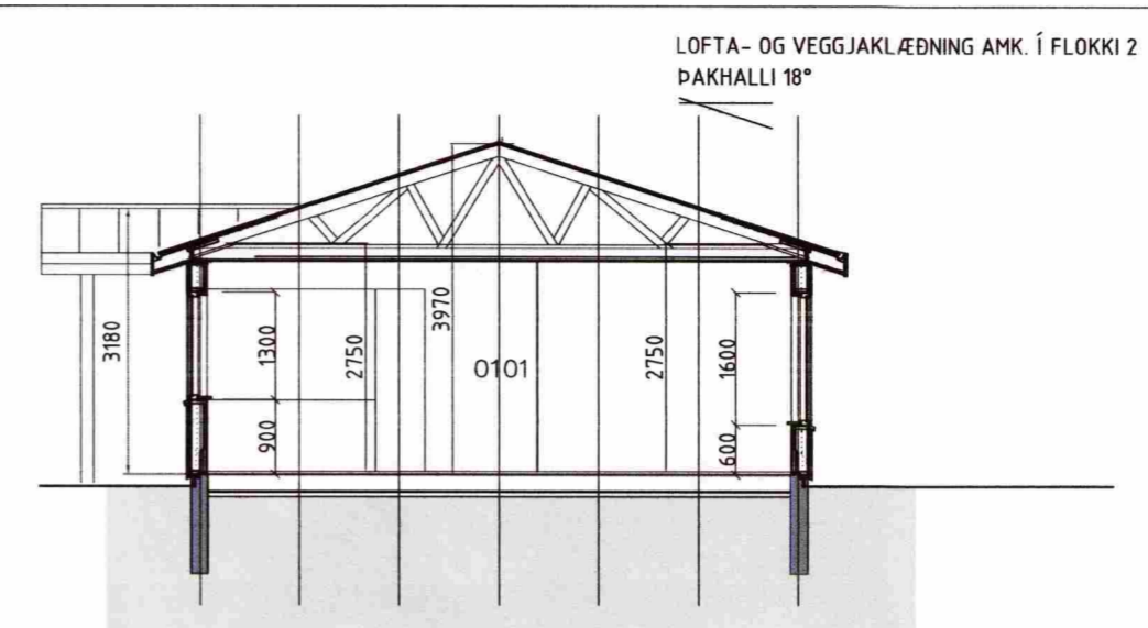
SNEIDMYND A-A
