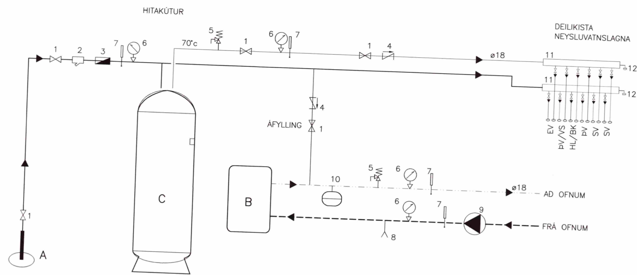
KERFISMYND HITA- OG NEYSLUVATNSKERFIS
