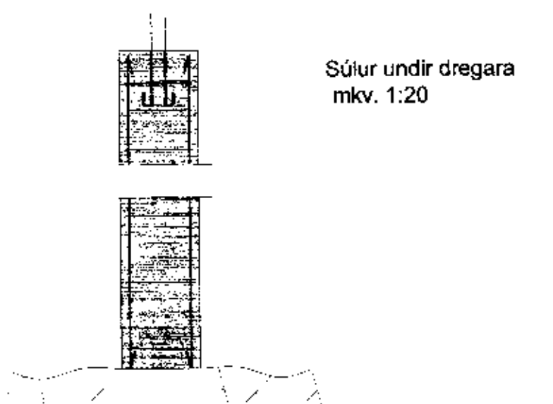
C Sneiðing 1:20
