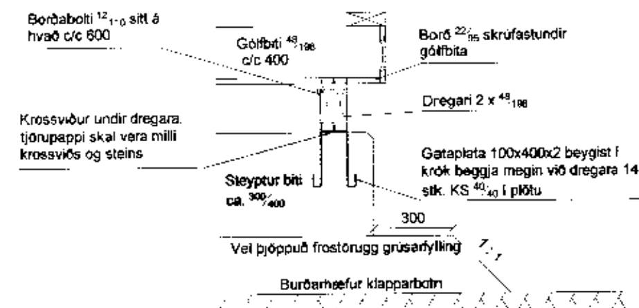
B Sneiðing 1:20
