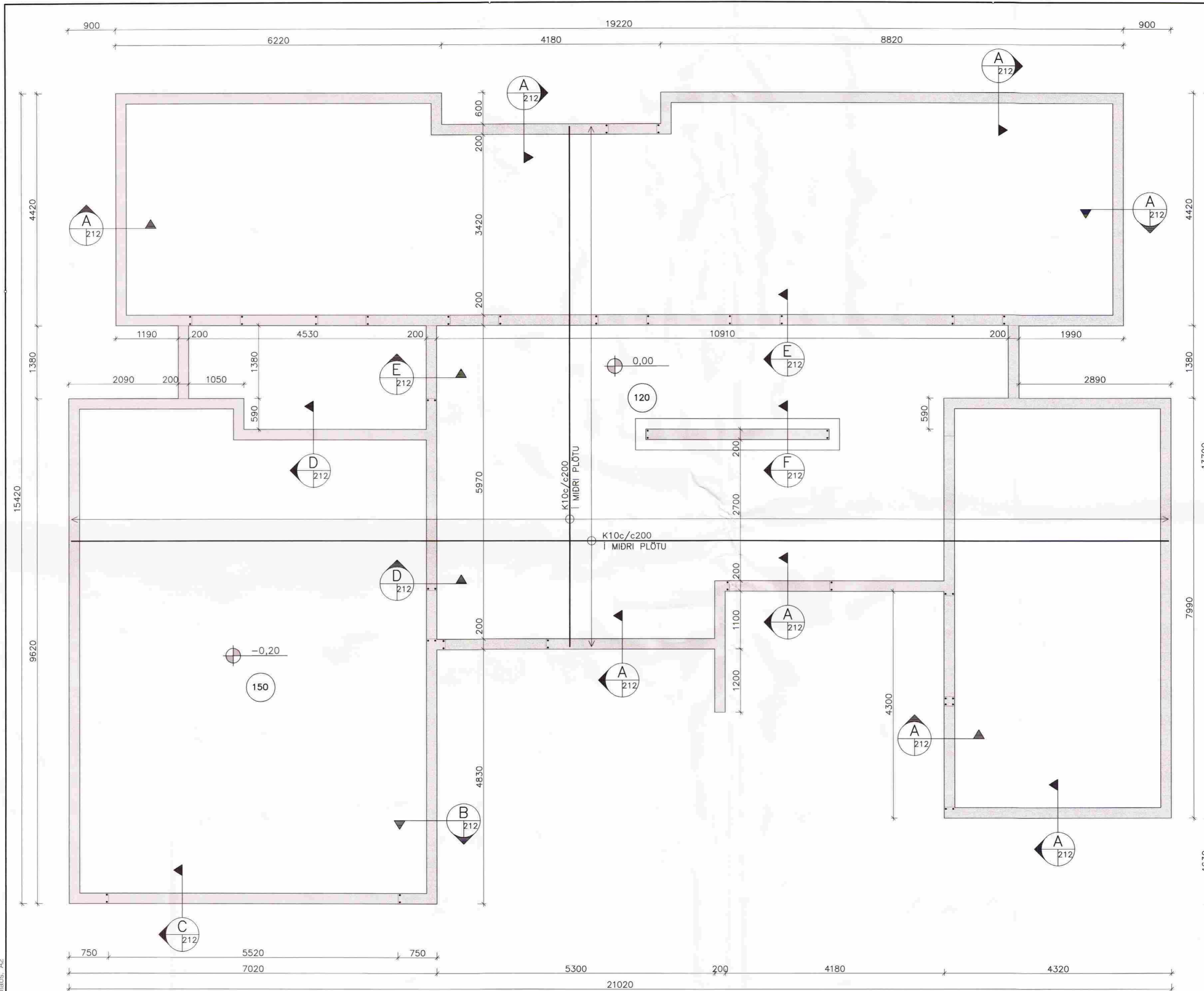
UNDIRSTÖÐUR –GRUNNMYND 1:50
