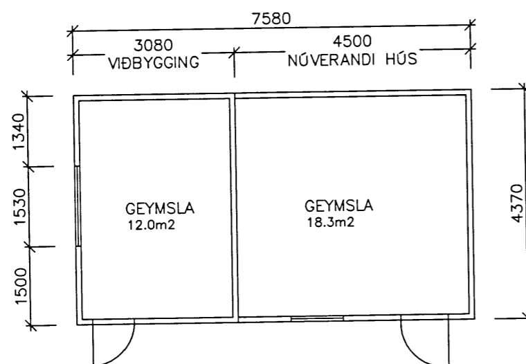
GRUNNMYND
