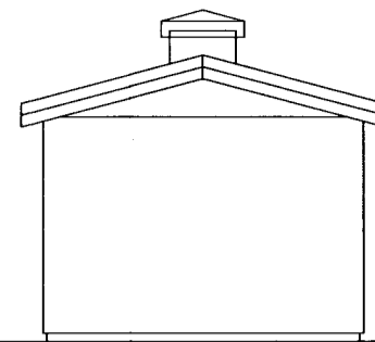
NORÐUR 1:100
