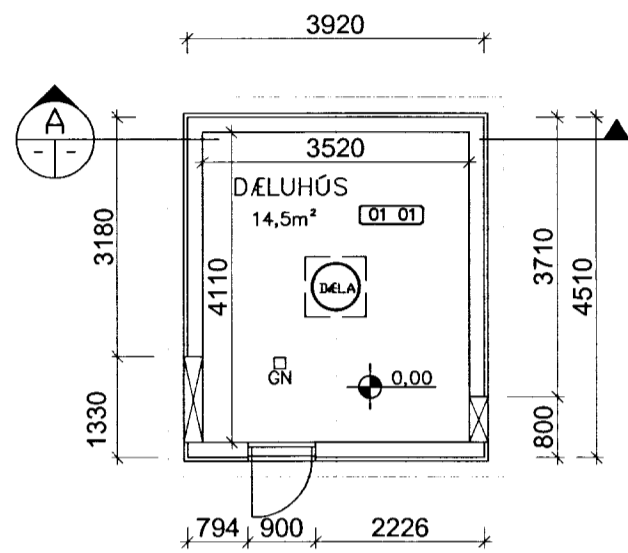
GRUNNMYND 1:100
