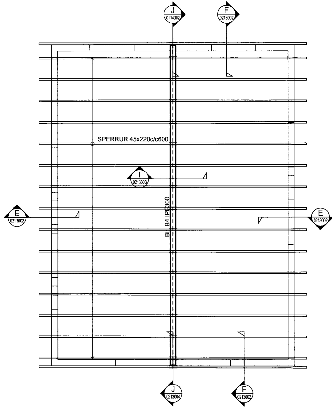
Bilgeymsla Grunnmynd - þakvirki M 1:50
