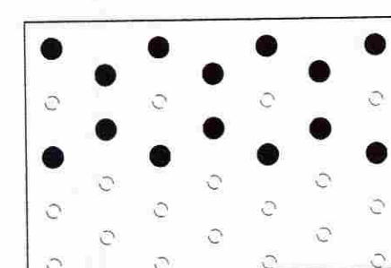
Negling í súlu/bita (nærri enda) 14 stk 40/50 kamsaumur
