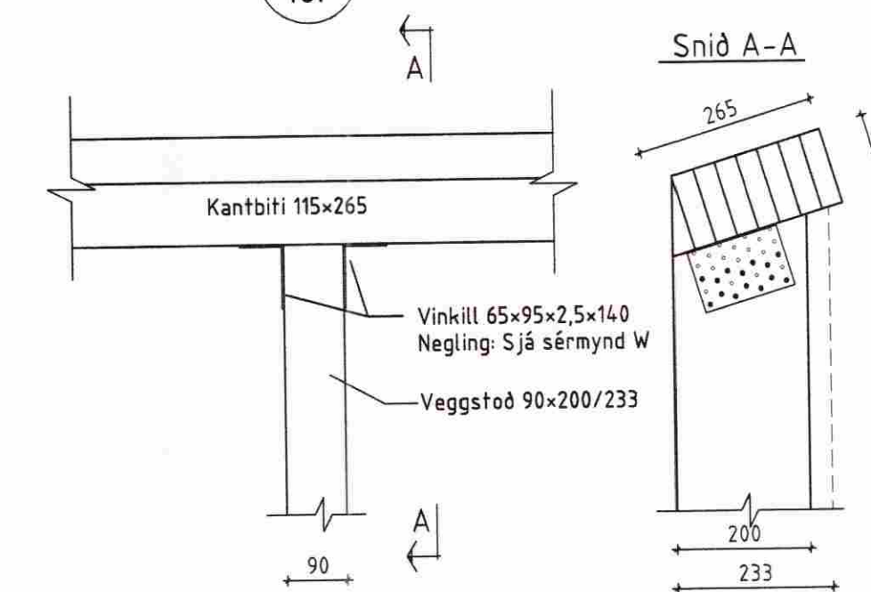
Sérmynd 24 Mkv.: 1:10
