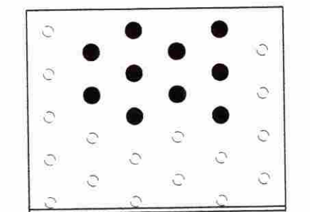
Negling í súlu/bita (nærri enda) 10 stk 40/50 kamsaumur
