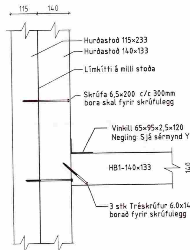
X - BMF-105 vinklar án st.
