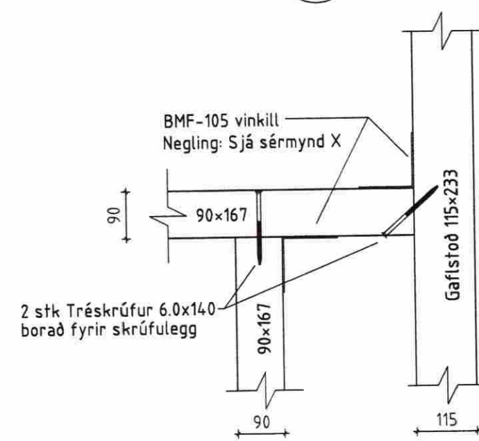
Sérmynd 22 Mkv.: 1:10
