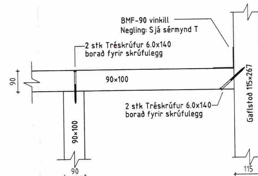
Sérmynd 23 Mkv.: 1:10
