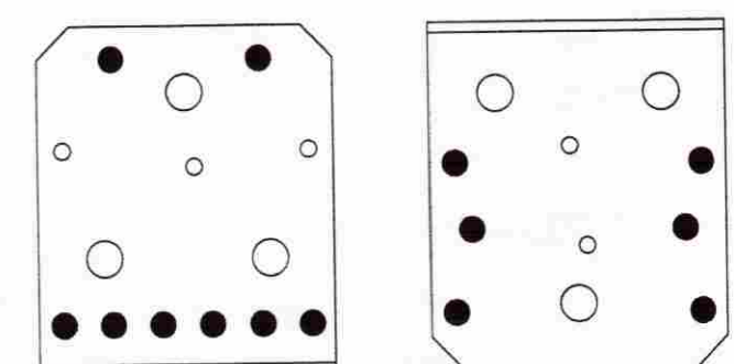
Negling í súlu/bita (fjarri enda) 8 stk 40/50 kamsaumur
