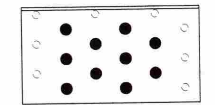
Negling í súlu/bita (fjarri enda) 10 stk 40/50 kamsaumur
