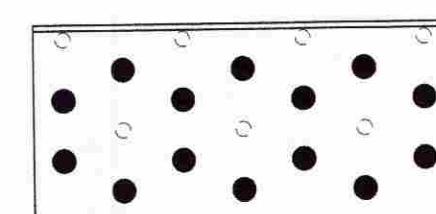
Negling í súlu/bita (fjarri enda) 14 stk 40/50 kamsaumur
