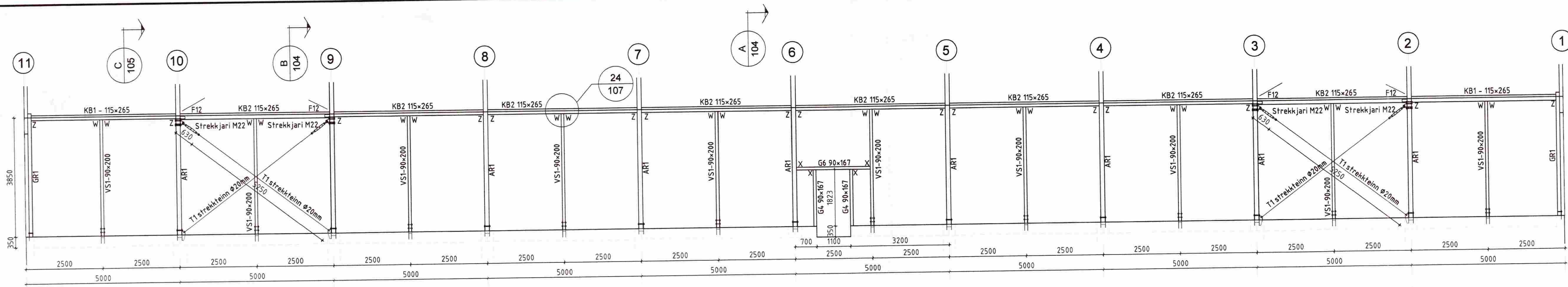
Ásýnd langhlíð Mkv. 1:75
