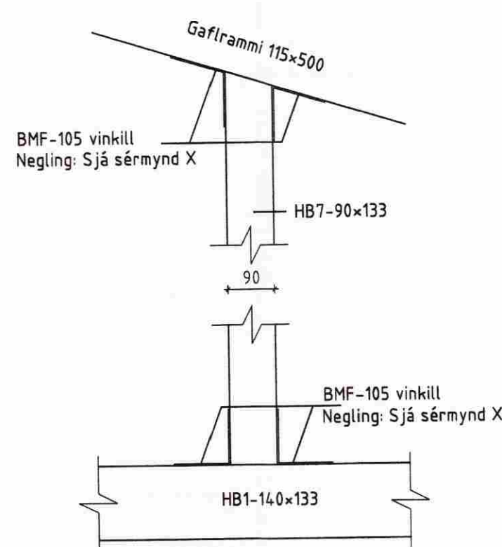
Sérmynd 21 Mkv.: 1:10
