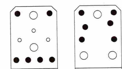
Negling í súlu/bita (fjarri enda) 6 stk 40/50 kamsaumur
