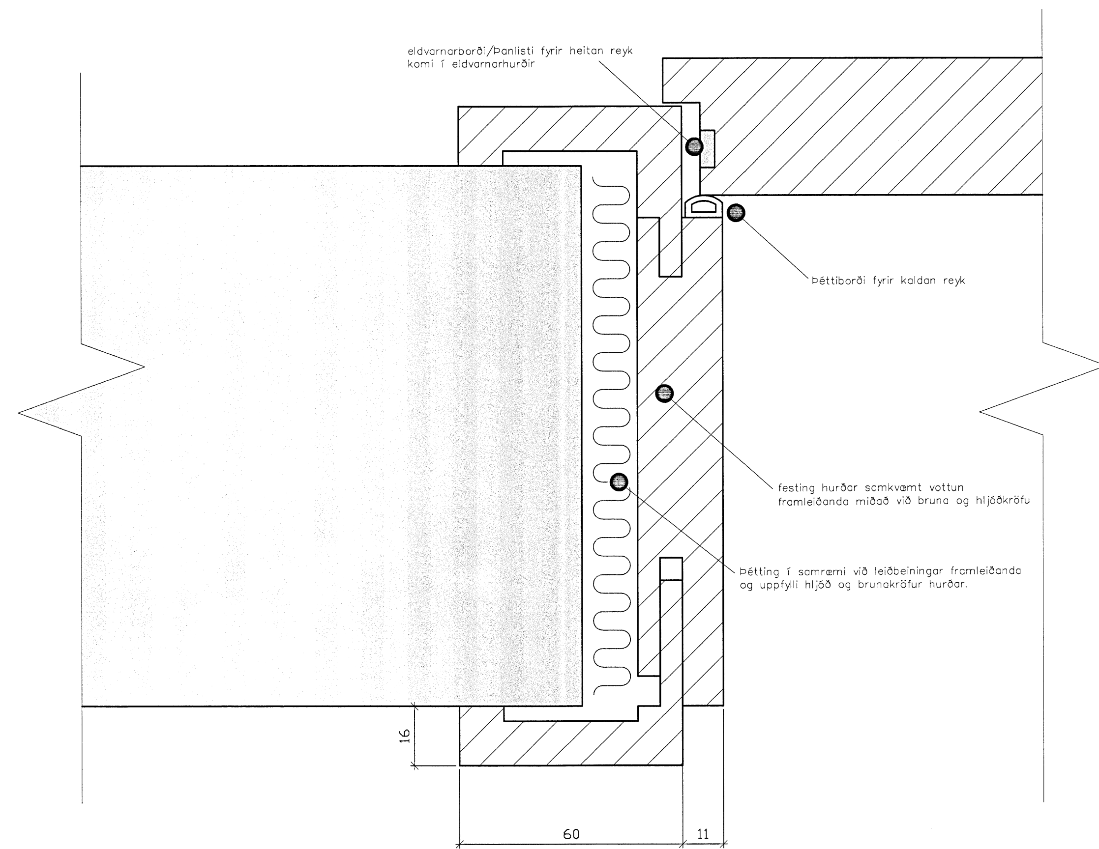
D frágangur, stöðluð yfirfelld hurð í steypnan vegg
