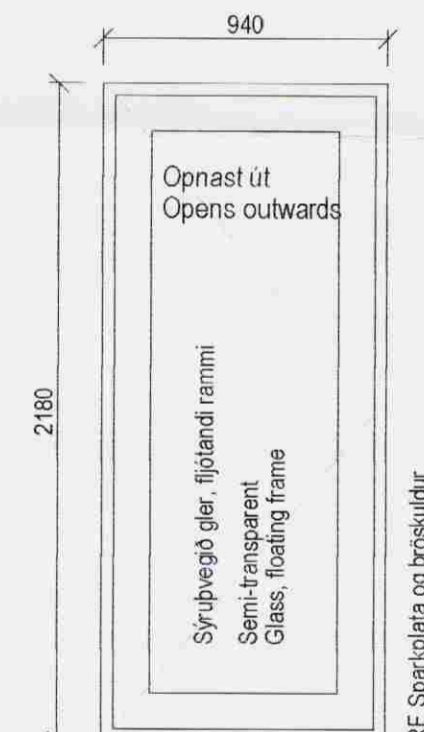
H-02, 2.stk M= 1:25
