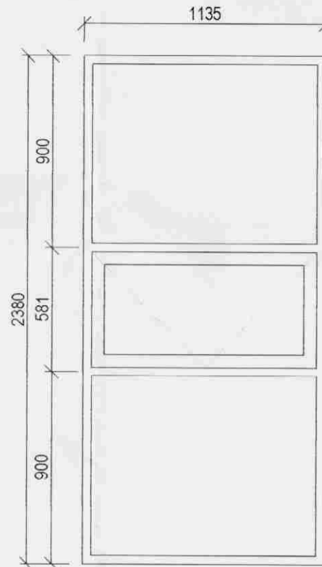
G-04, 2.stk M= 1:25
