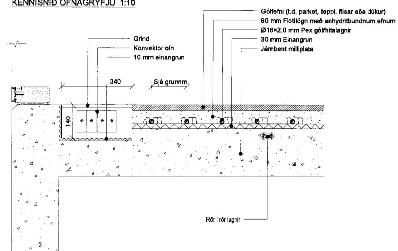
KENNISNIÐ OFNAGRYFJU 1:10
