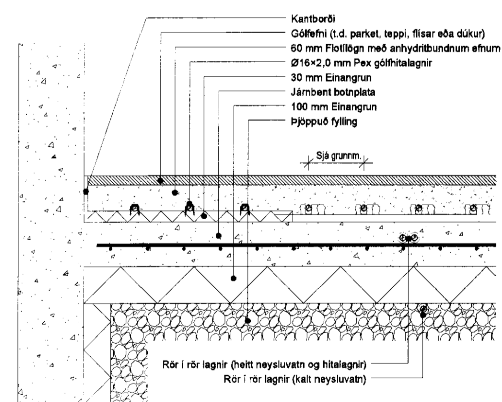
KENNISNIÐ GÓLFHITA 1:10
