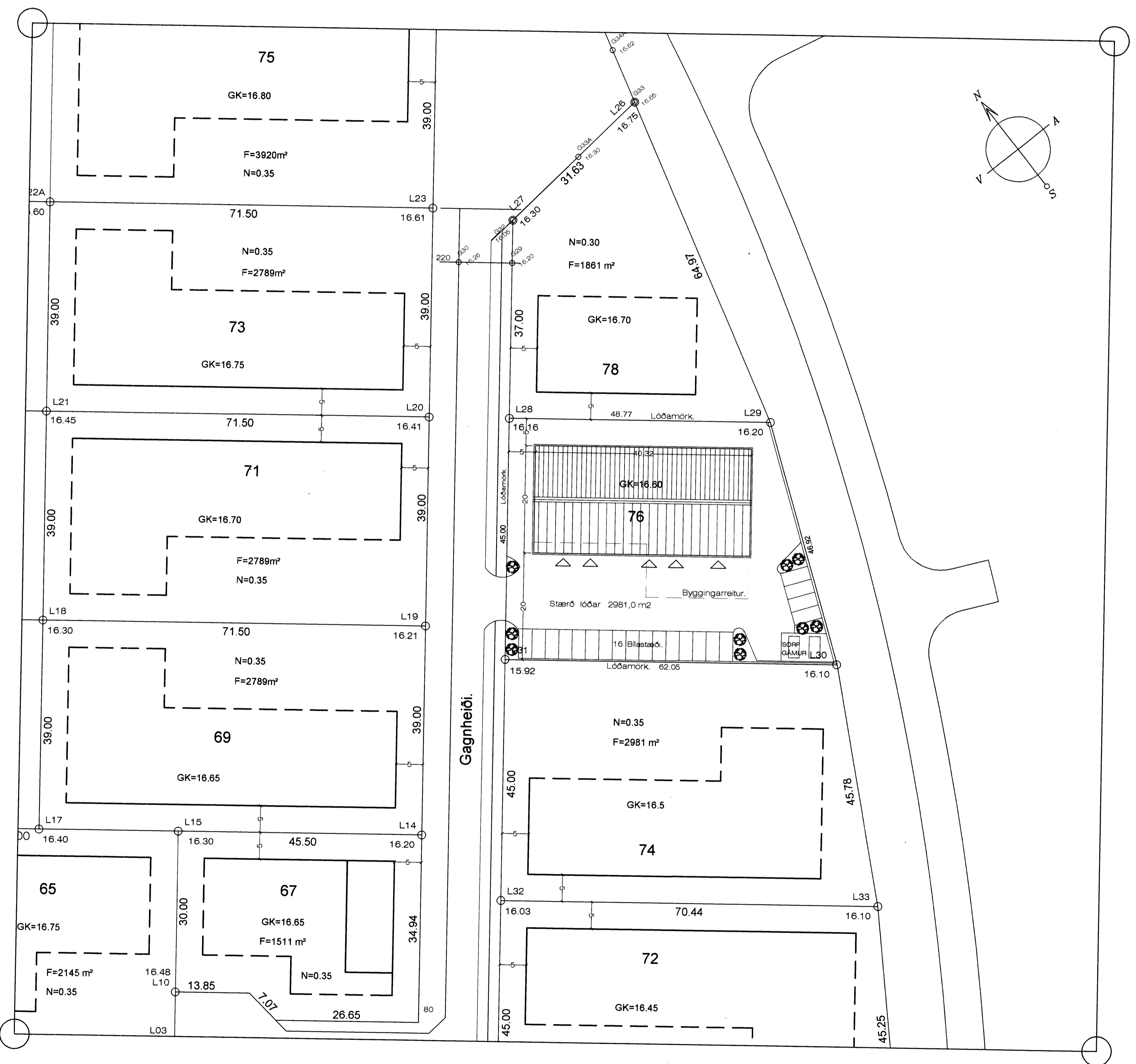
AFSTÖÐUMYND. 1:500
