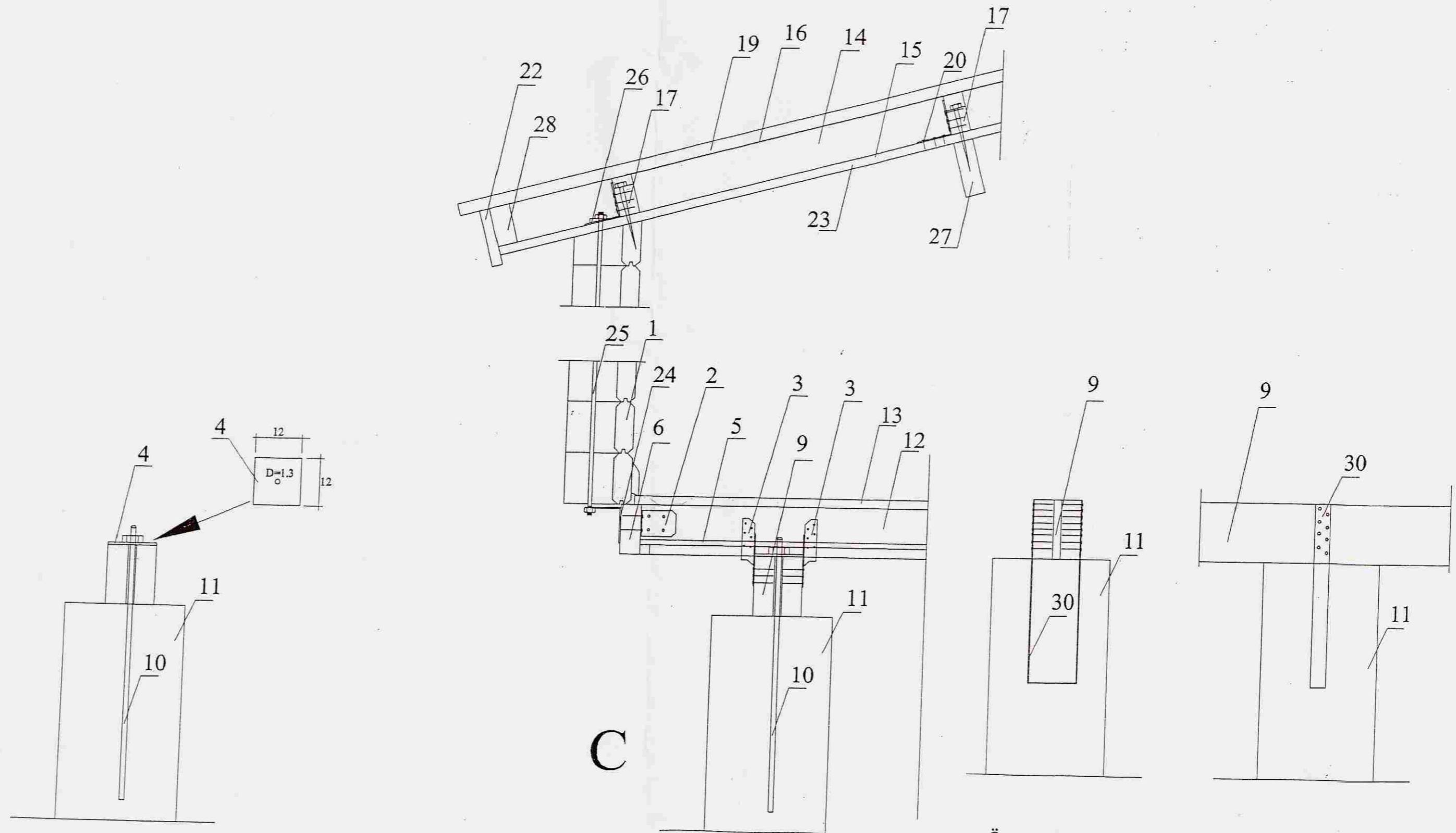
Önnur útgáfa af festingu húss við steypa súlu
