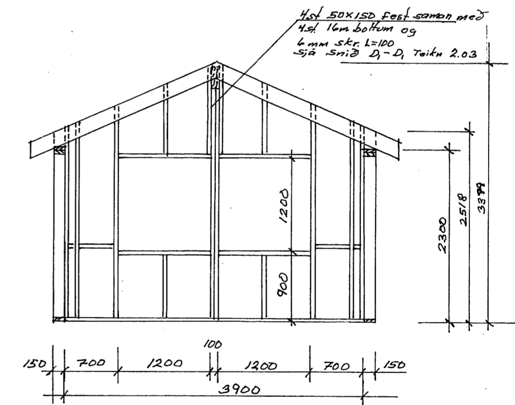
Veggur V4 M = 1:50
