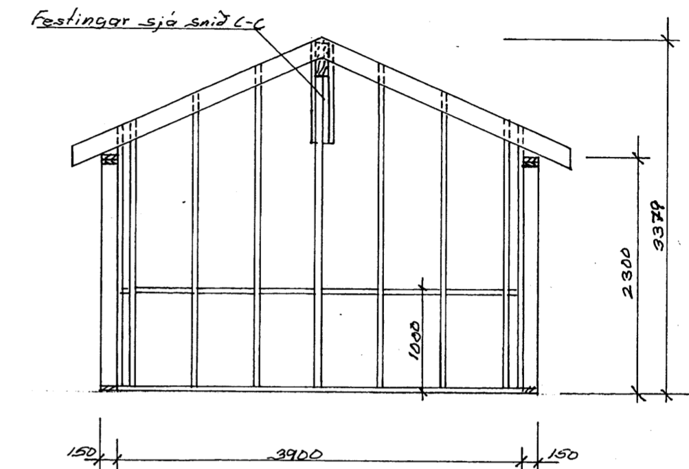
Veggur V2 M = 1:50
