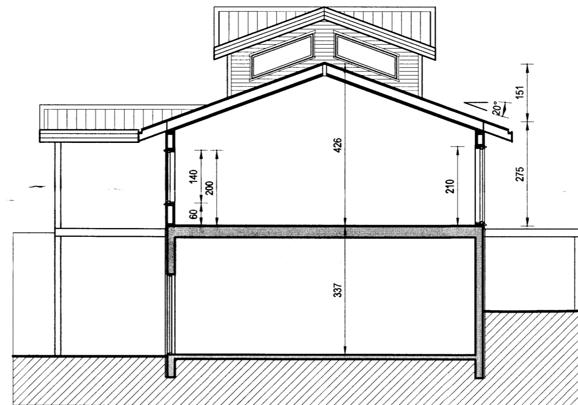
SNID A-A
