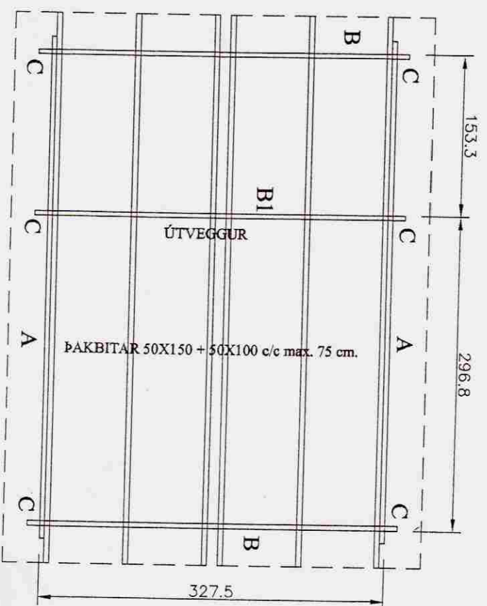
Grunnmynd þak
