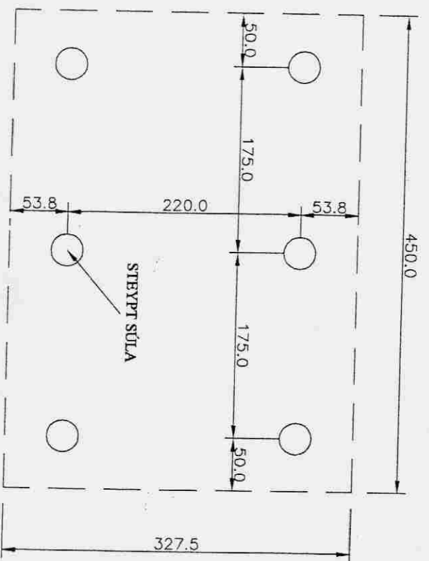
Grunnmynd steyptar súlu
