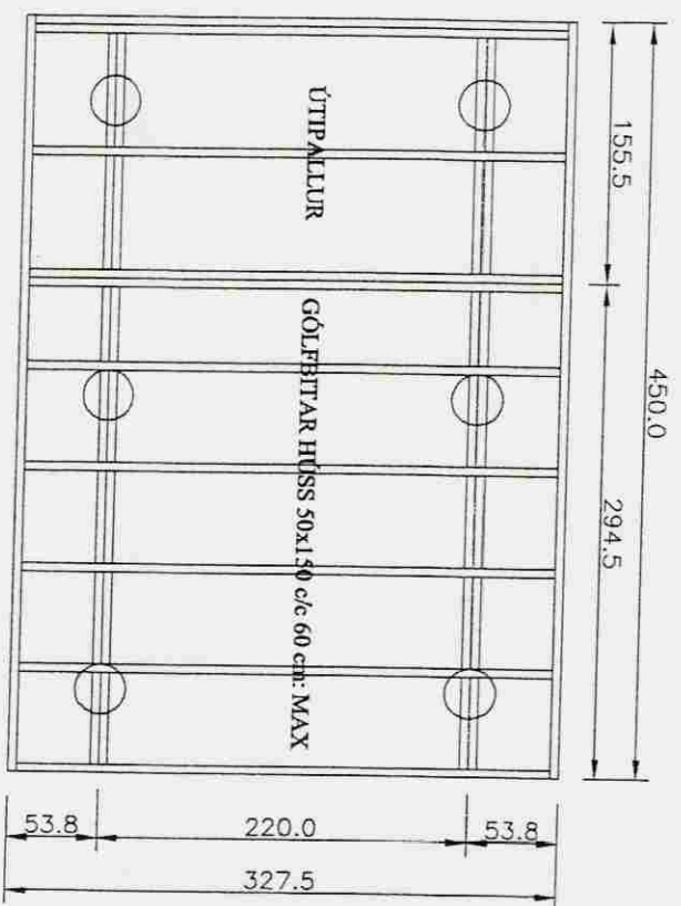
Grunnmynd gólfbitar
