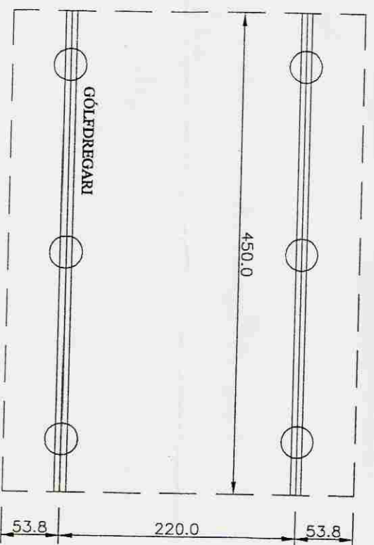
Grunnmynd dregarar
