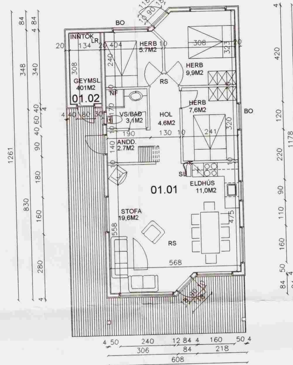
GRUNNMYND
