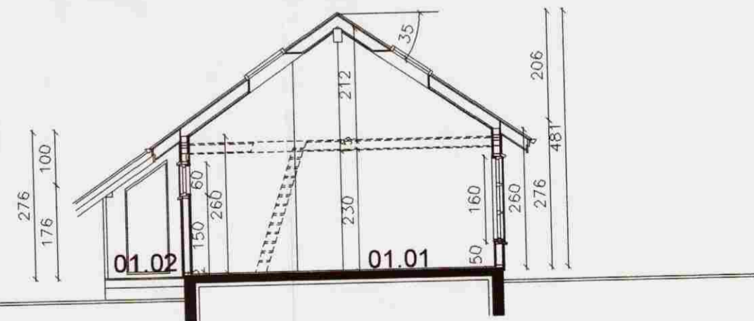
SKURÐUR A.
