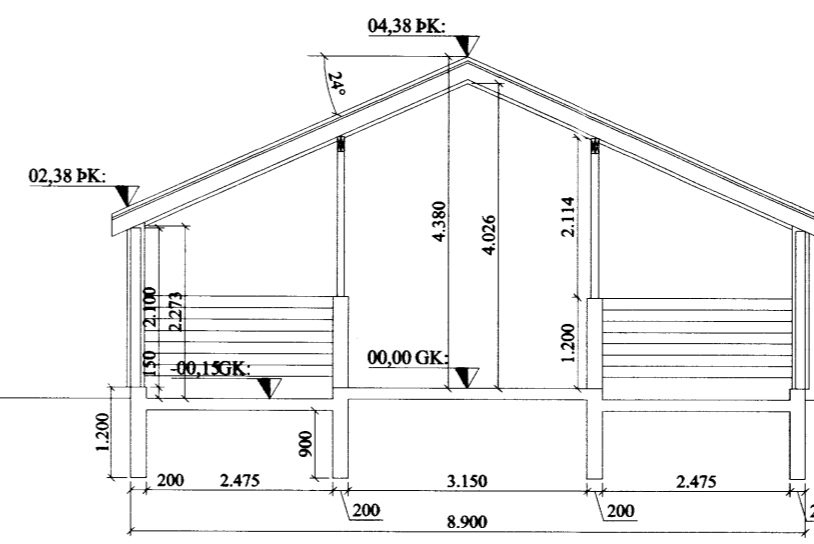
Snið C-C
