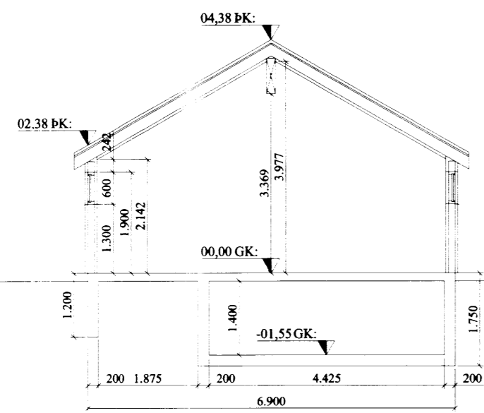
Snið A-A
