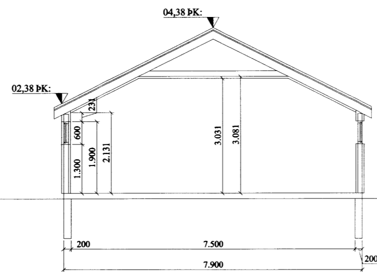
Snið B-B
