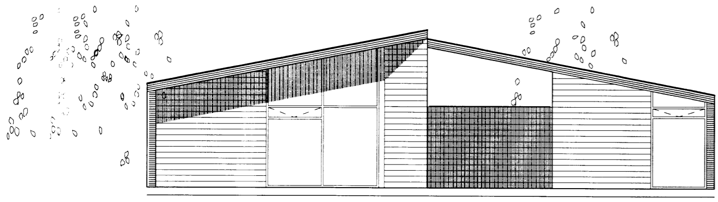
VESTUR ÚTLIT
