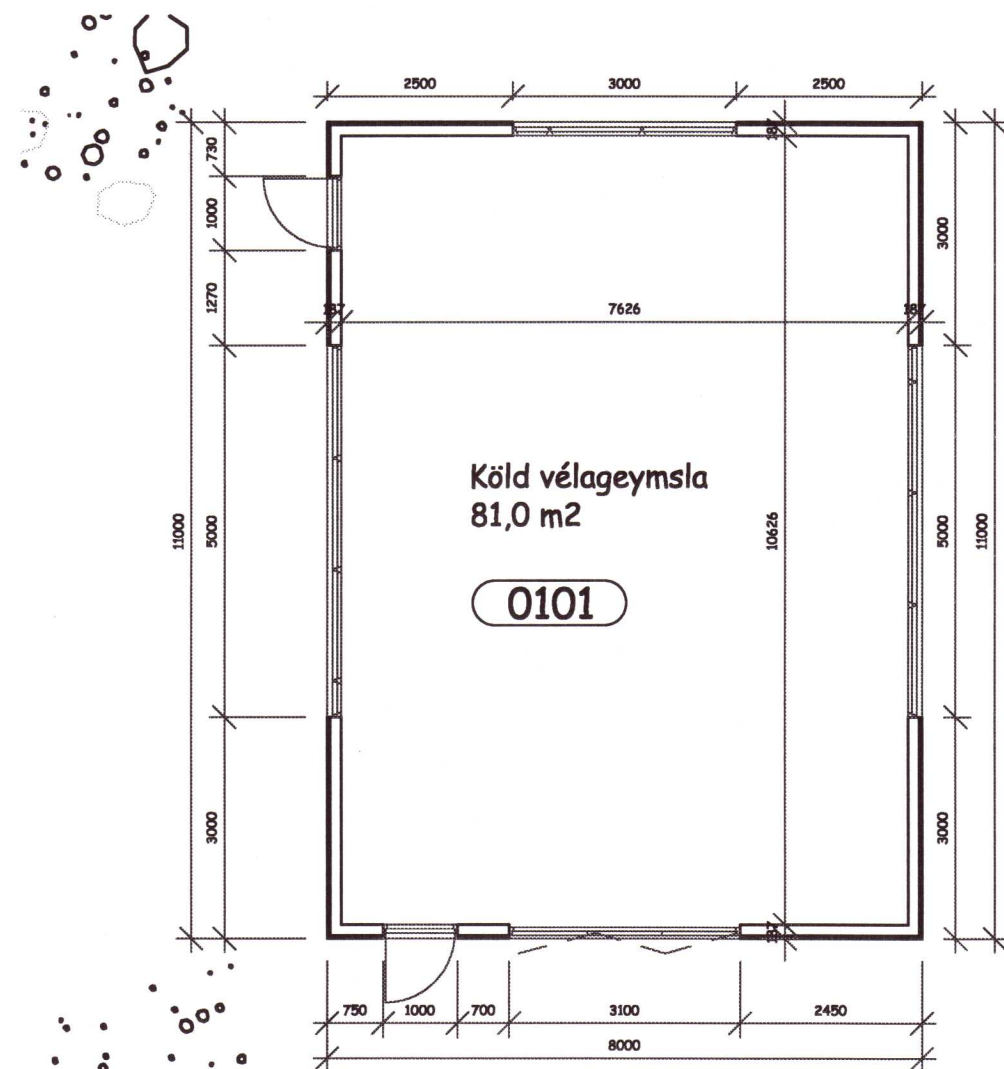
GRUNNMYND mkv. 1:100
