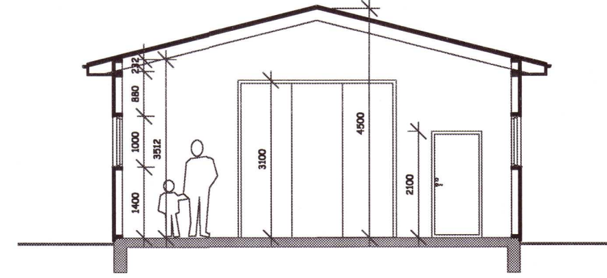
SNEIÐING mkv. 1:100
