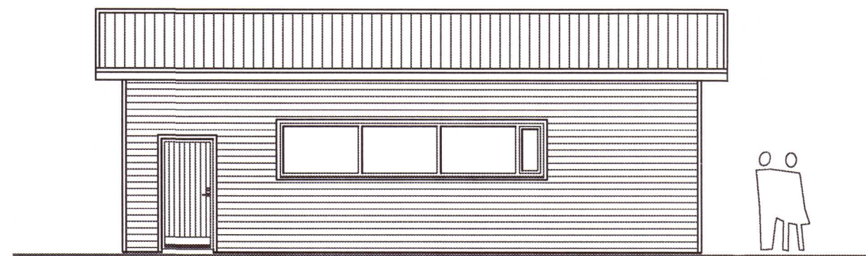
ÚTLIT VESTUR mkv. 1:100
