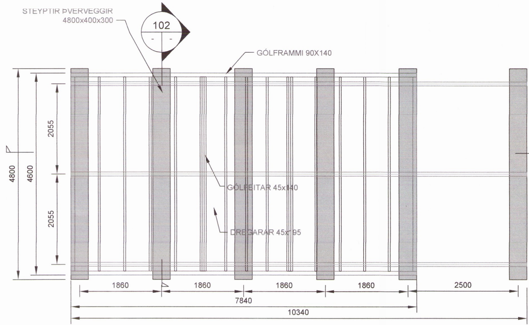
GRUNNMYND-UNDIRSTÖÐUR MKV. 1:50
