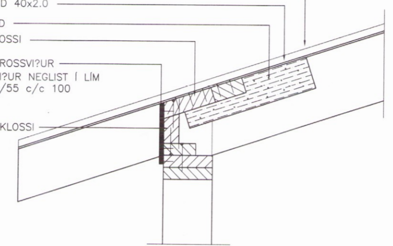
SNID B-B MKV. 1:10
