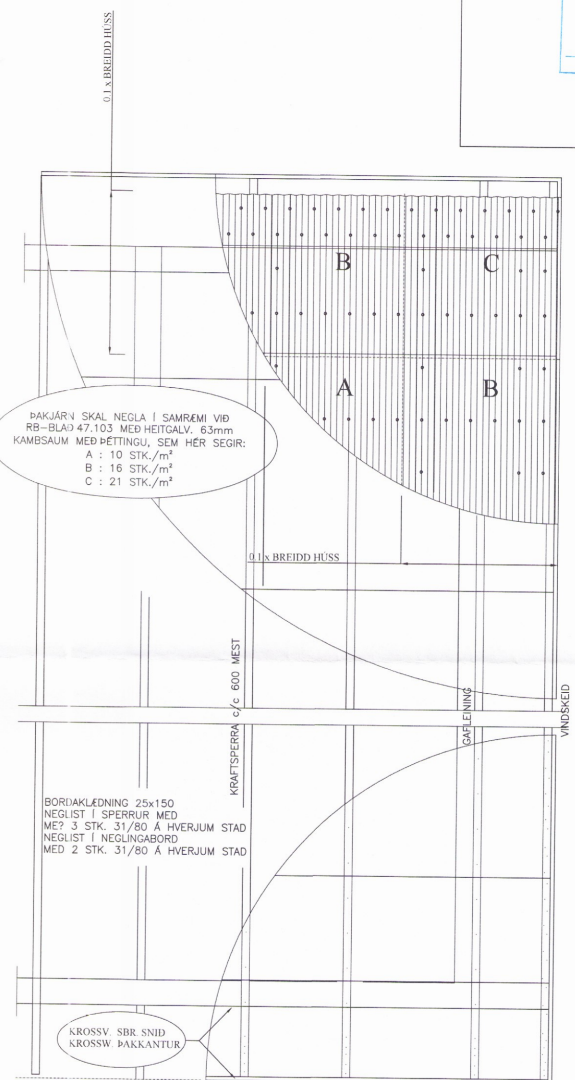
NEGLING ÞAKKLÉÐNINGAR MKV. 1:20
