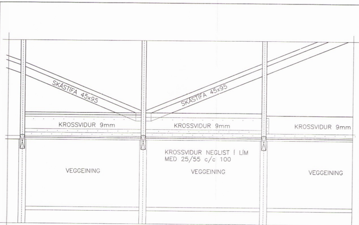
HLIÐARMYND MKV. 1:20
