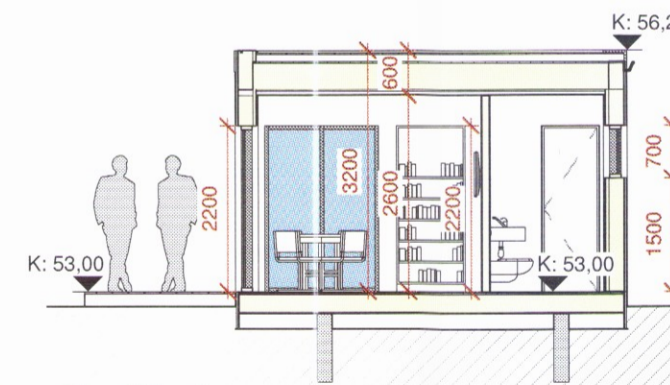
6 Snið 1 1 : 100
