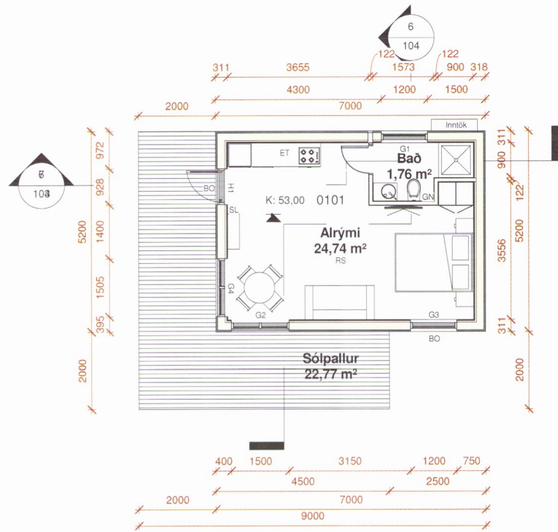
1 Húsagerð 1 1 : 100
