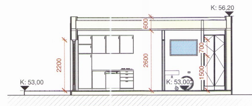
7 Snið 2 1 : 100
