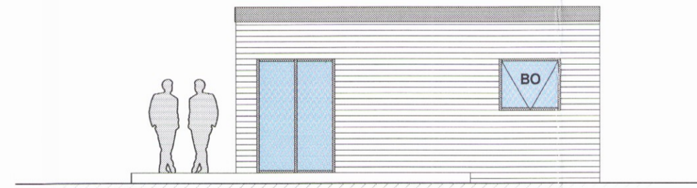
4 Suð-Austur - 2 1 : 100
