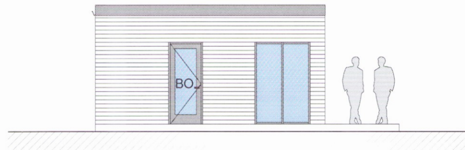
3 Suð-Vestur - 2 1 : 100
