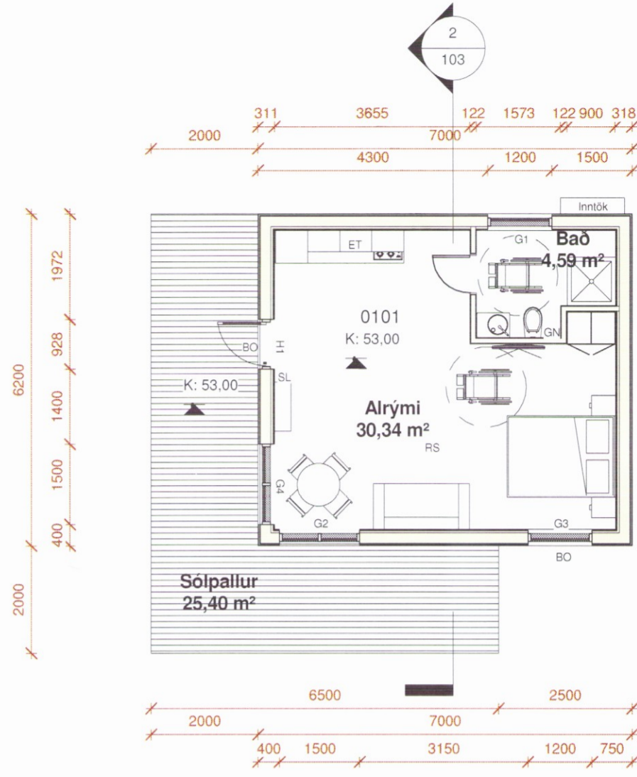
1 Húsagerð 2 1 : 100
