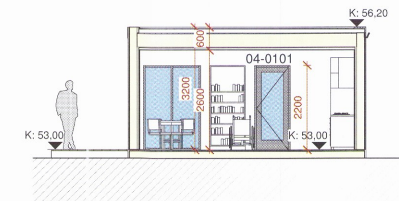
2 Snið 3 - B 1 : 100
