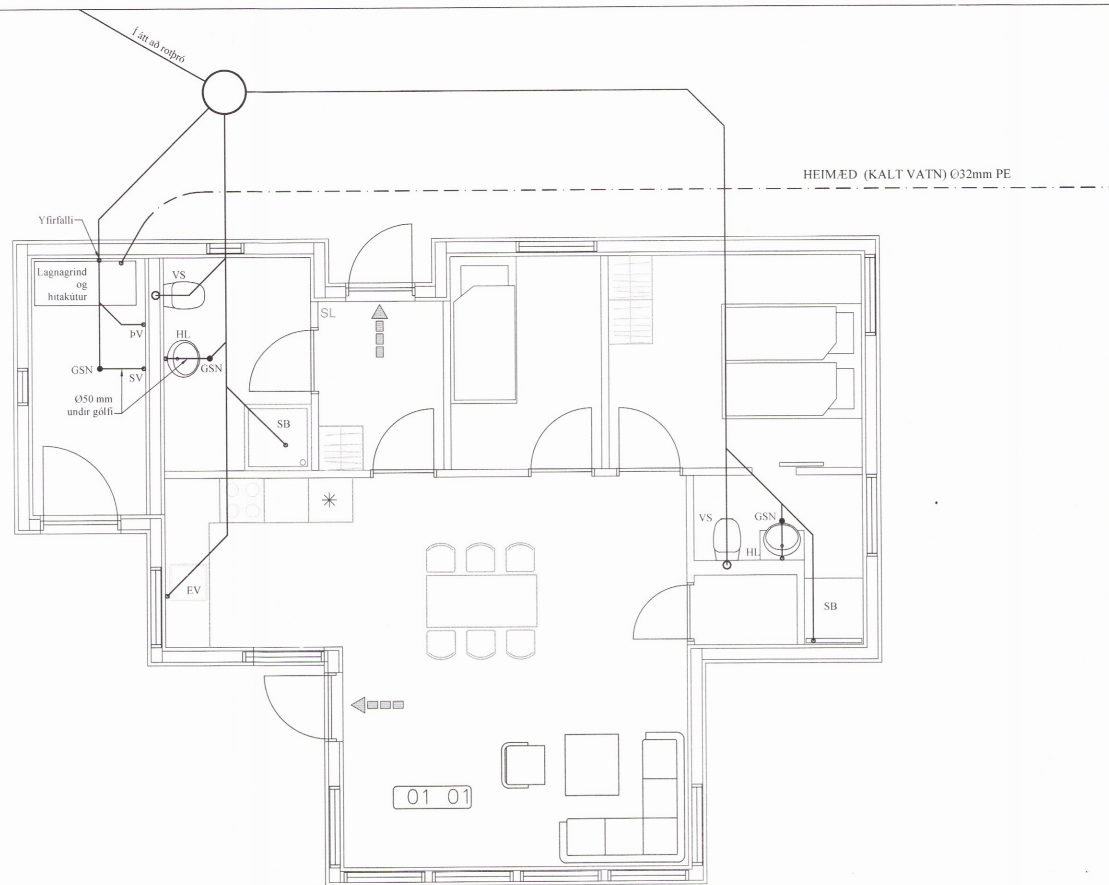
GRUNNMYND FRÁRENNSLISLAGNA Mkv. 1:50
