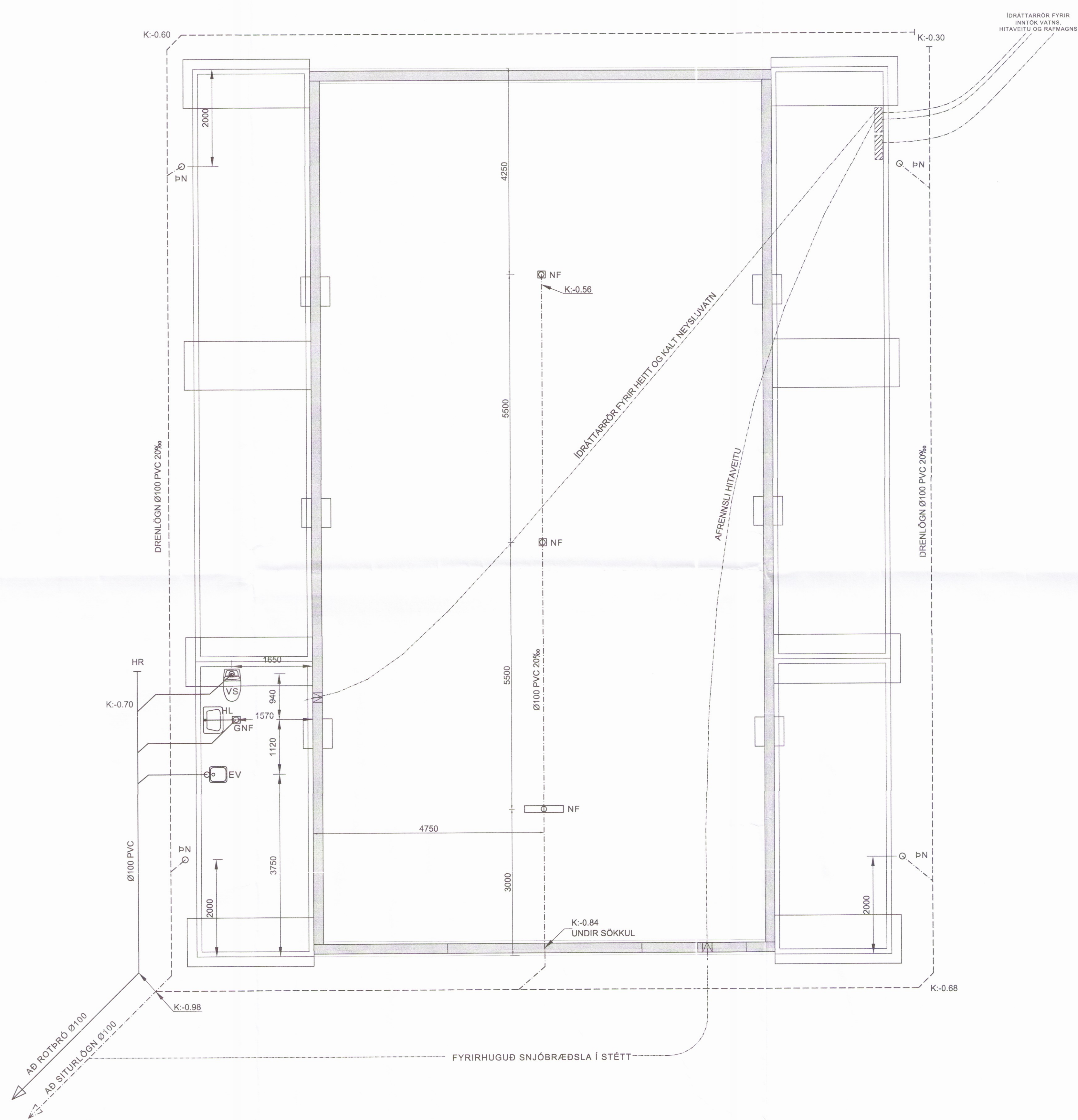
GRUNNMYND GRUNNLAGNIR MKV. 1:50
