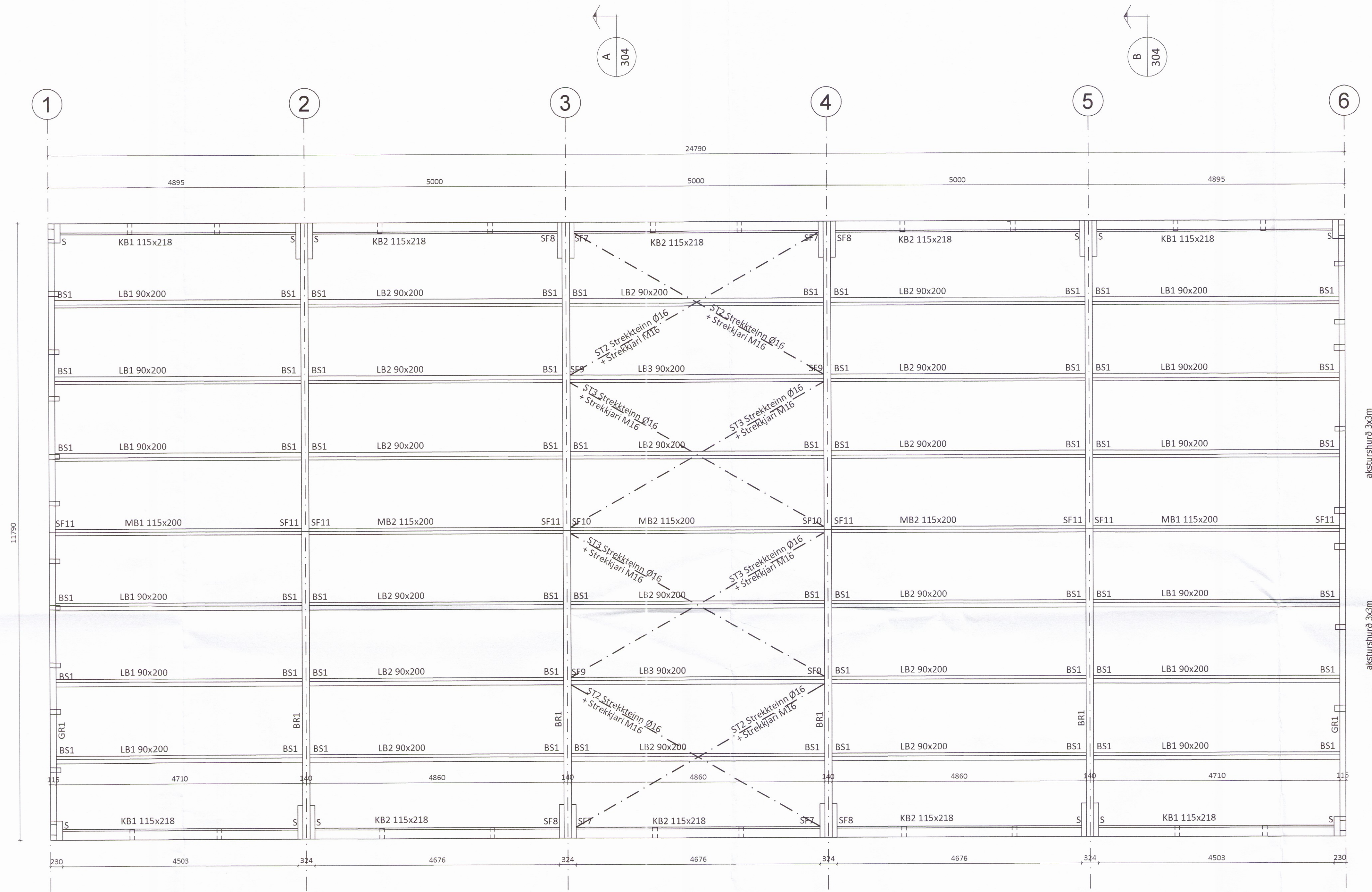
Þakmynd Mkv. 1:50
