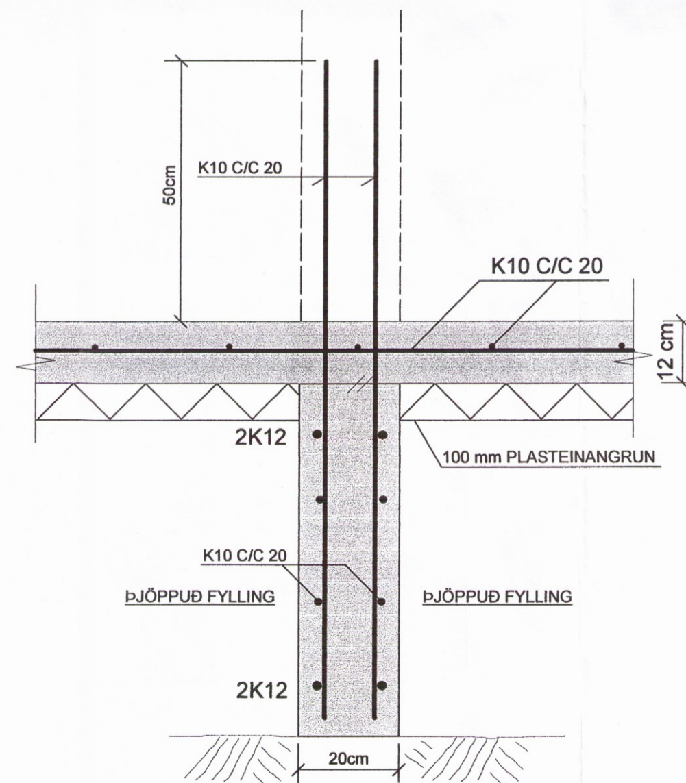
SNIÐ E-E MKV. 1:10
