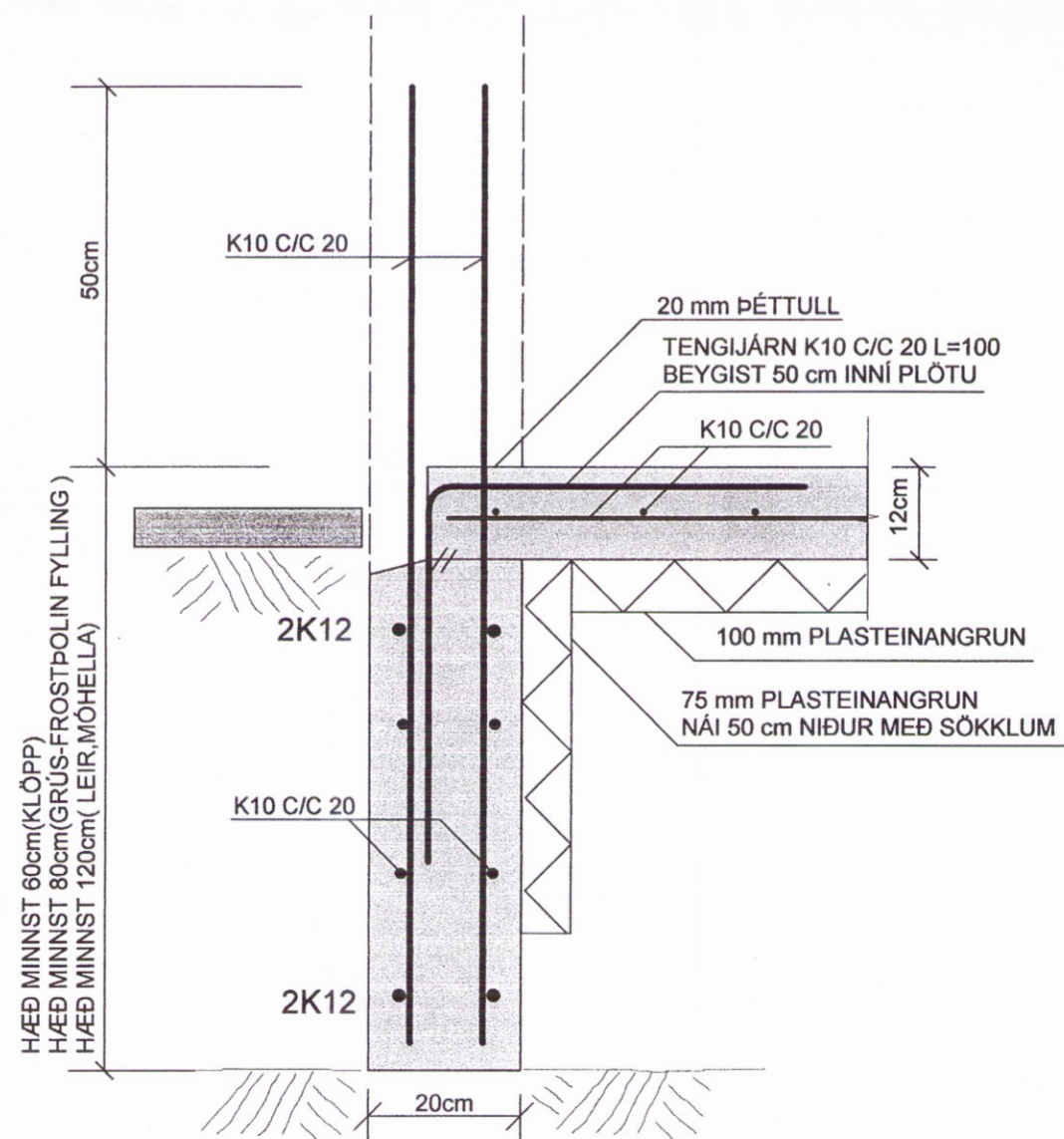
SNIÐ D-D MKV. 1:10
