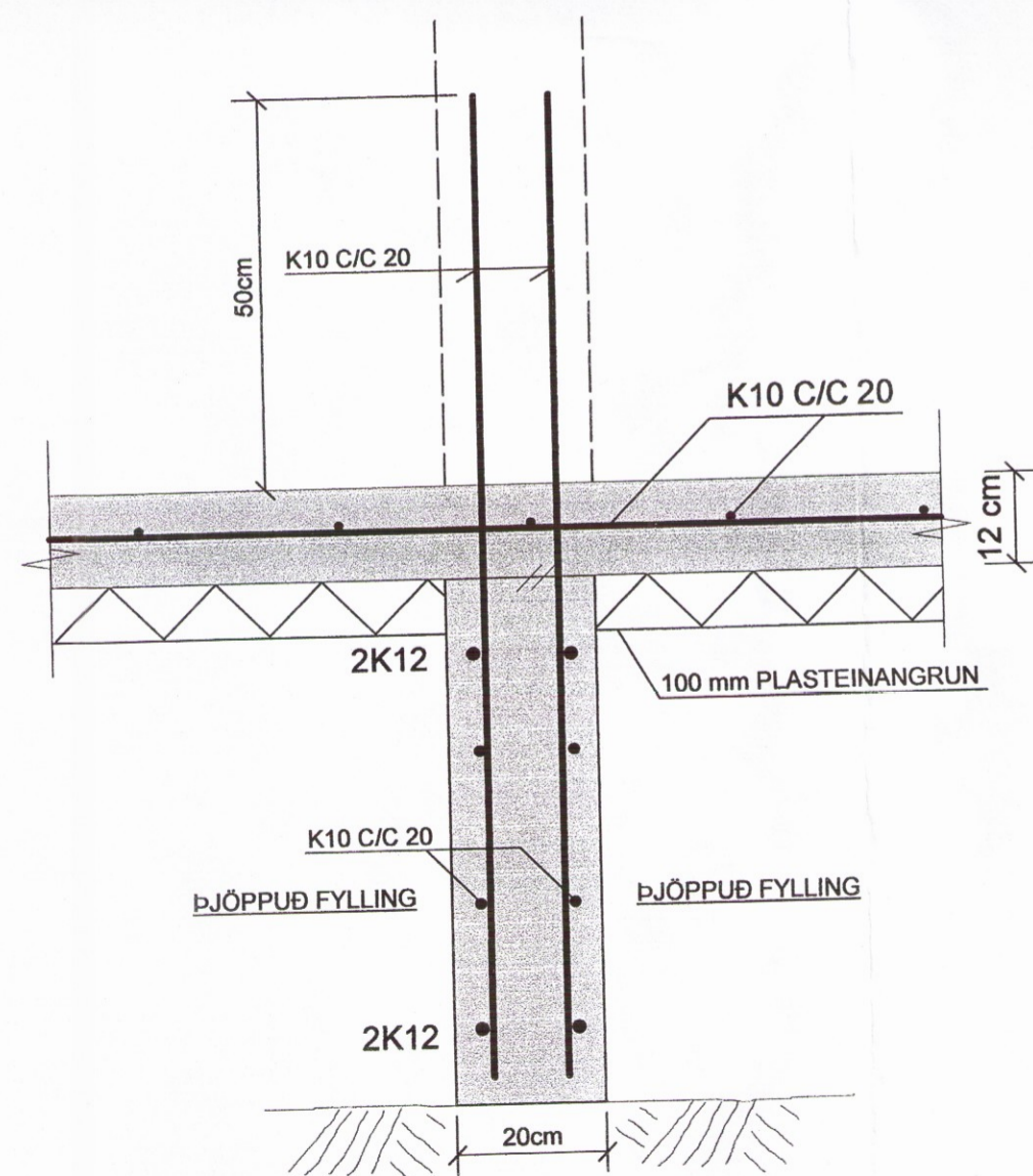
SNID E-E MKV. 1:10
