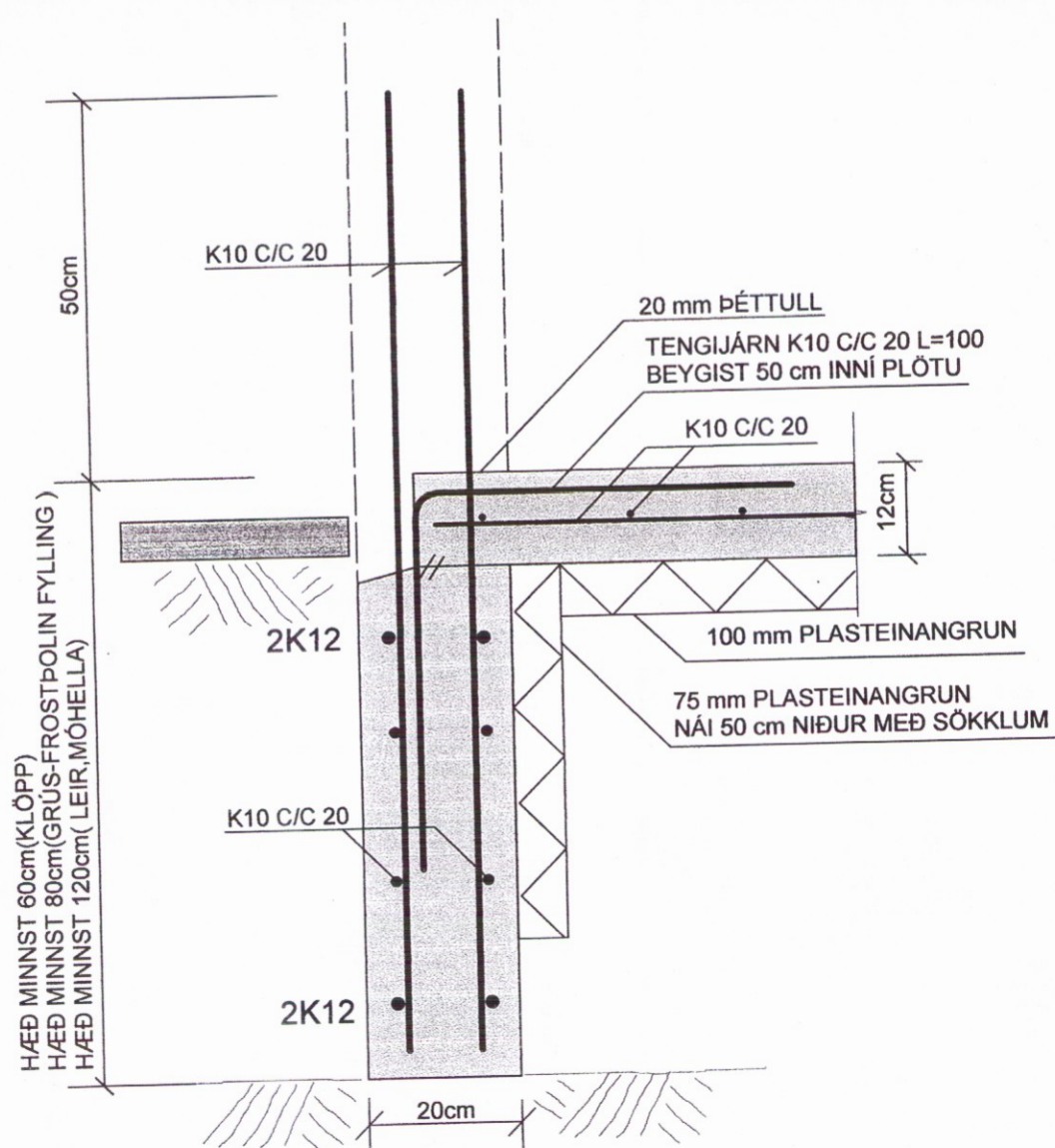
SNID D-D MKV. 1:10
