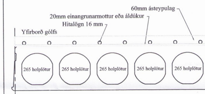
Útfærsla á hitalögnum í milliplötu
