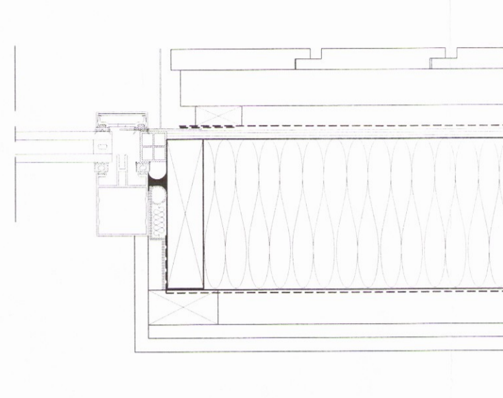
D.6 Gluggar/ALMENNT. MKV 1:5
