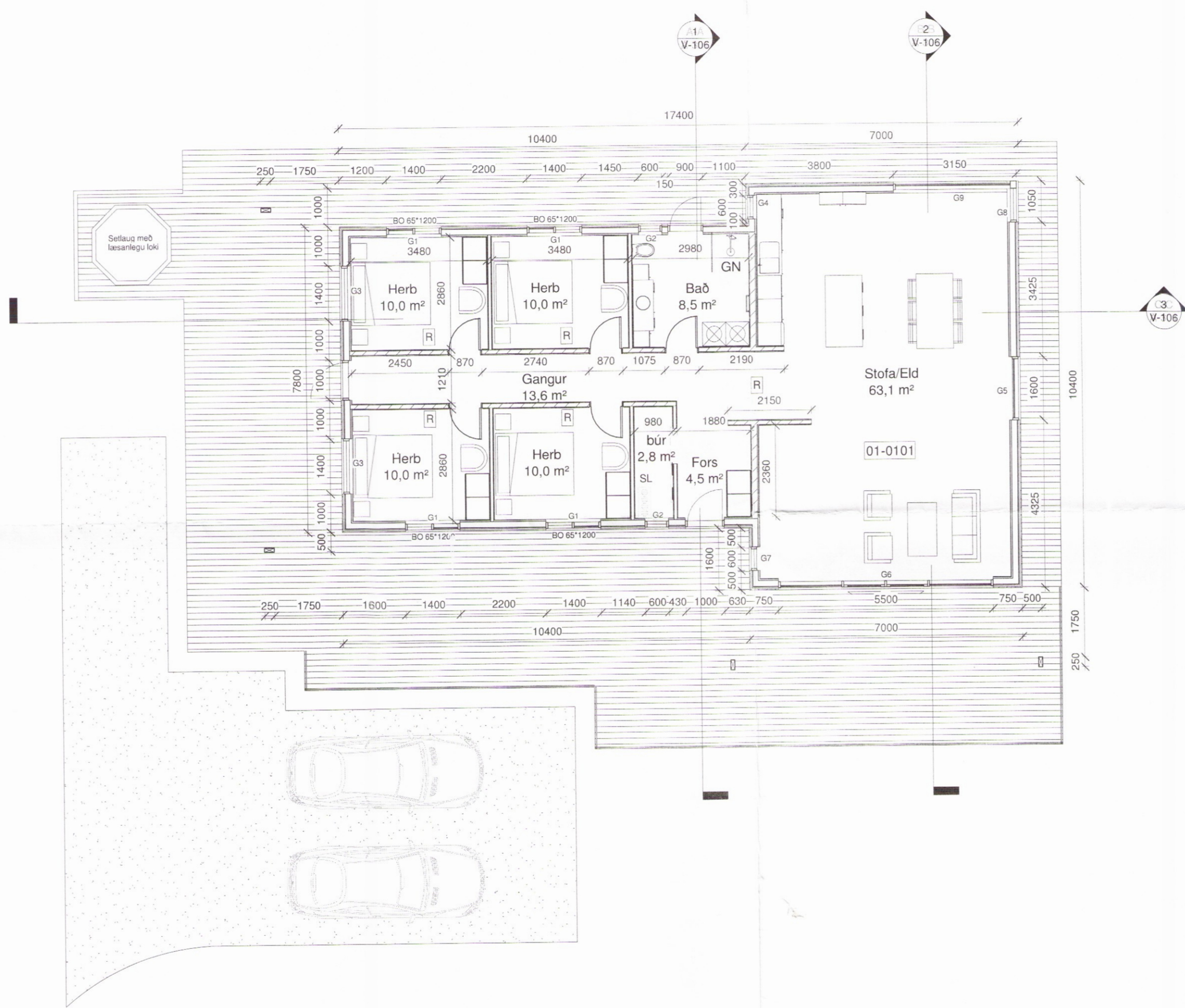
Grunnmynd 1 hæð 1 : 100
