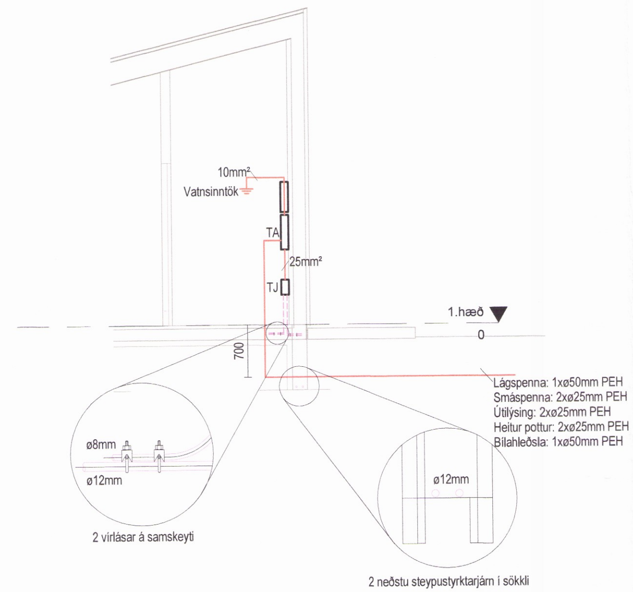
Snið í inntök - Hús 17 1 : 50
