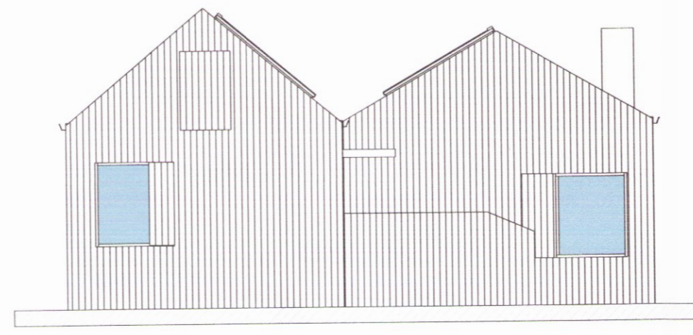
Suður 1 : 100
