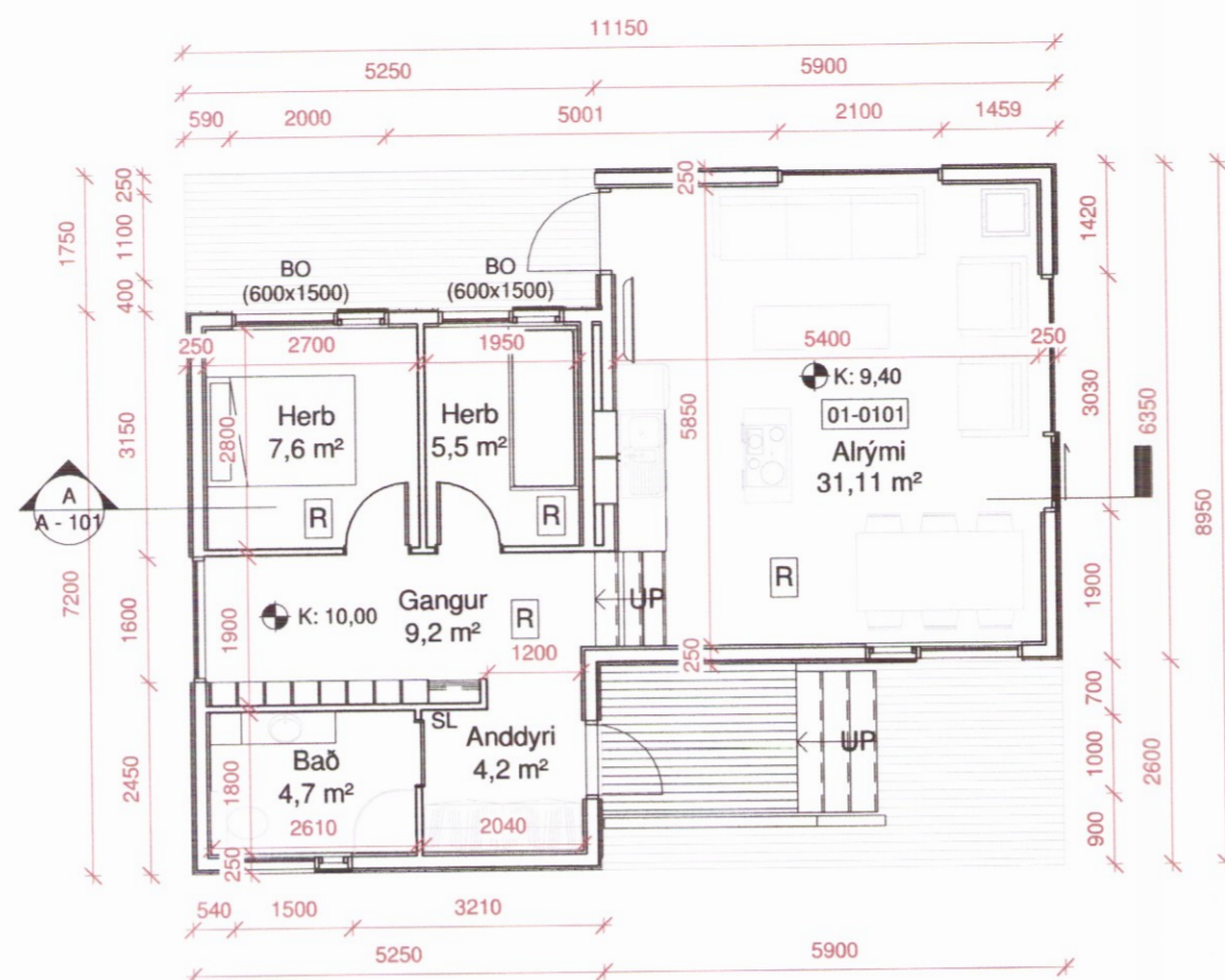
Grunnmynd 1 : 100
