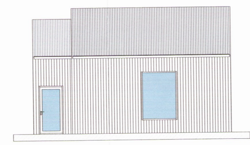
Vestur 1 : 100
