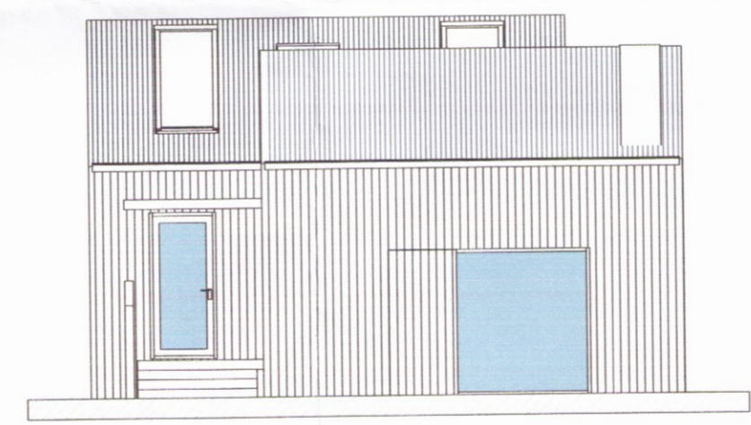
Austur 1 : 100
