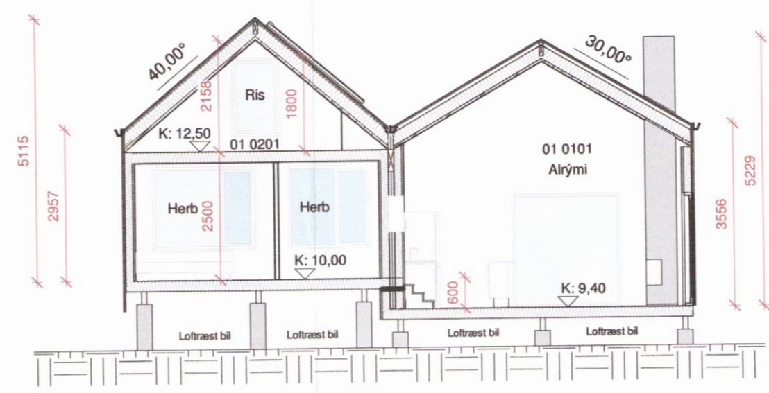
Sneiðing A-A 1 : 100
