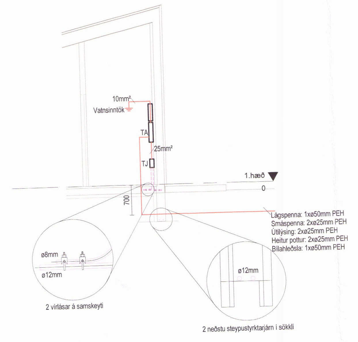
Snið í inntök 1 : 50
