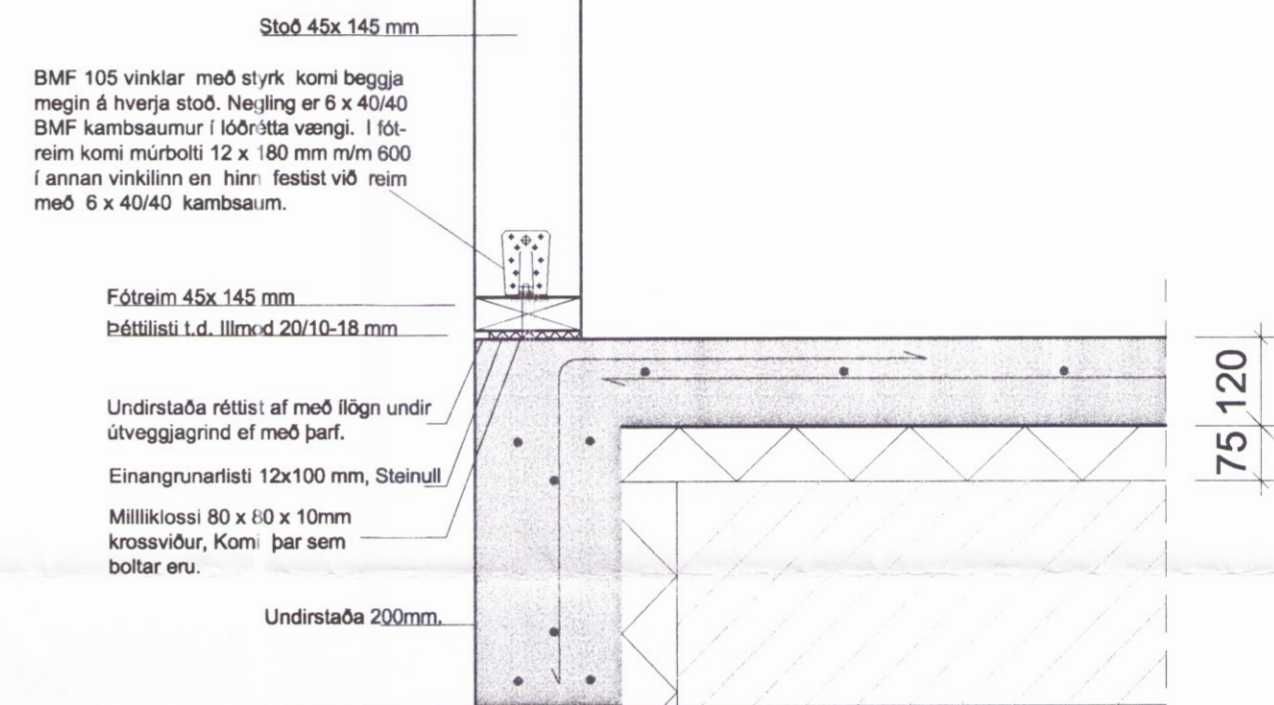
B Snið í enda, timburgrind Mkv. 1:10
