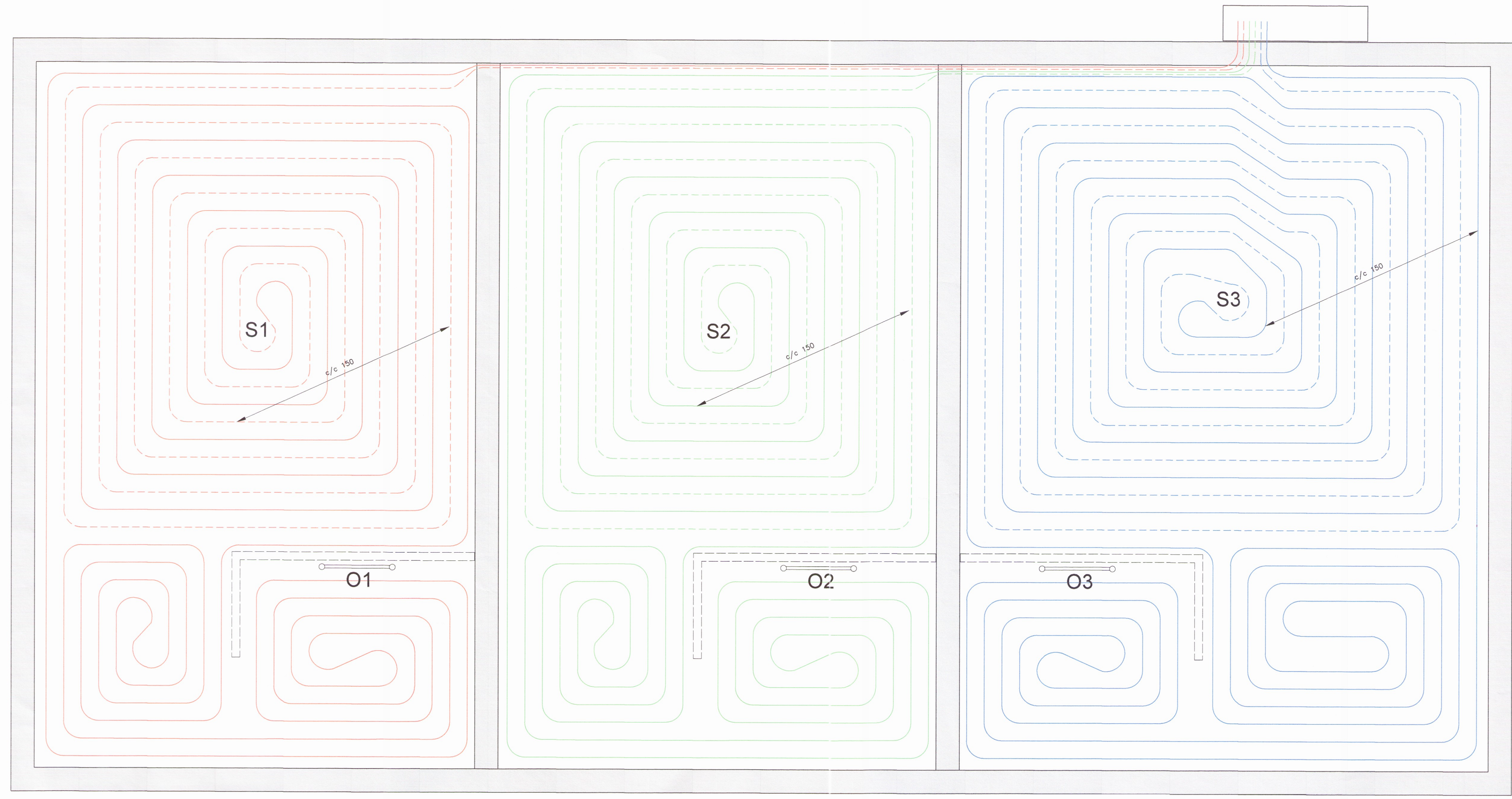
GRUNNMYND HITALAGNIR MKV. 1:20
