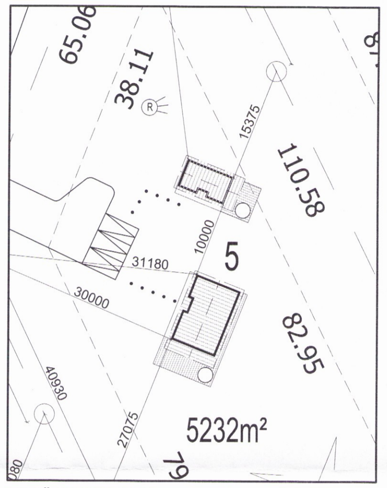
AFSTÖÐUMYND 1:500
