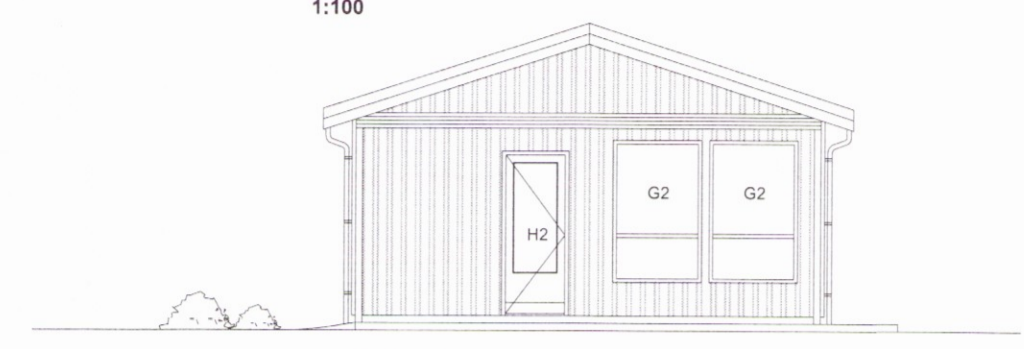
ÚTLIT SUÐUR 1:100
