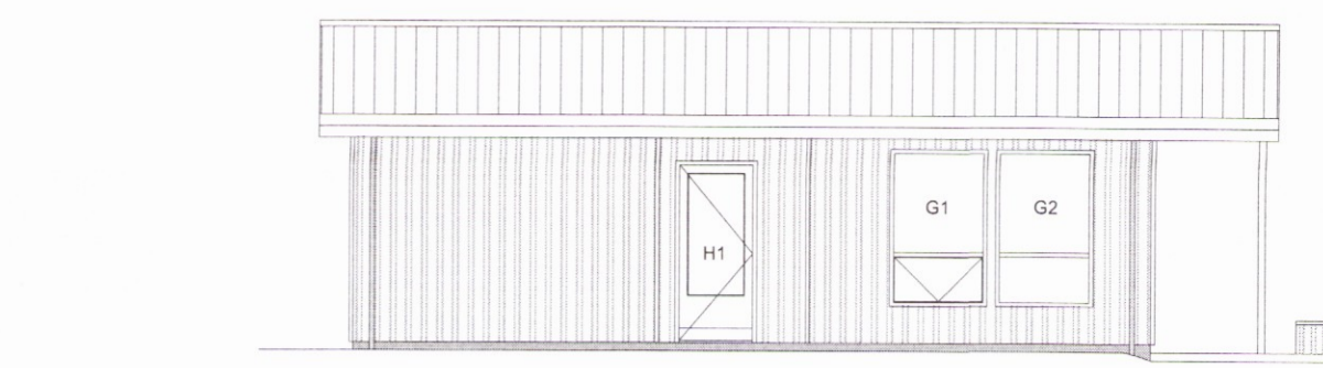
ÚTLIT VESTUR 1:100
