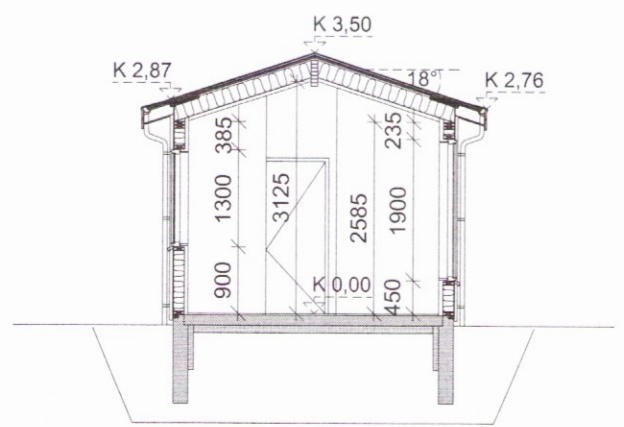
SNIÐ A-A 1:100
