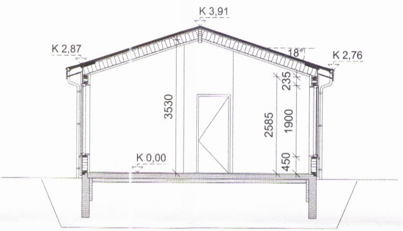
SNIÐ A-A 1:100
