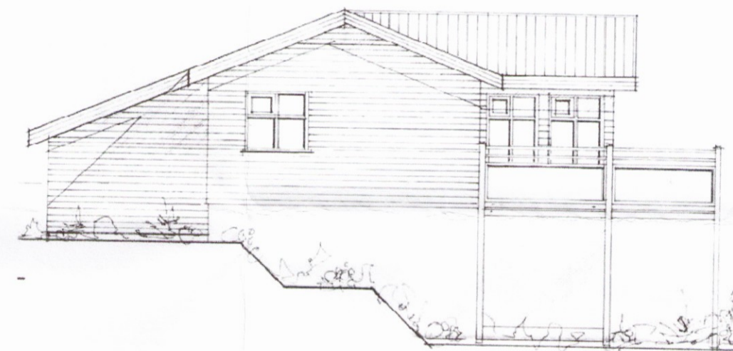
Útlit vestur 1:100
