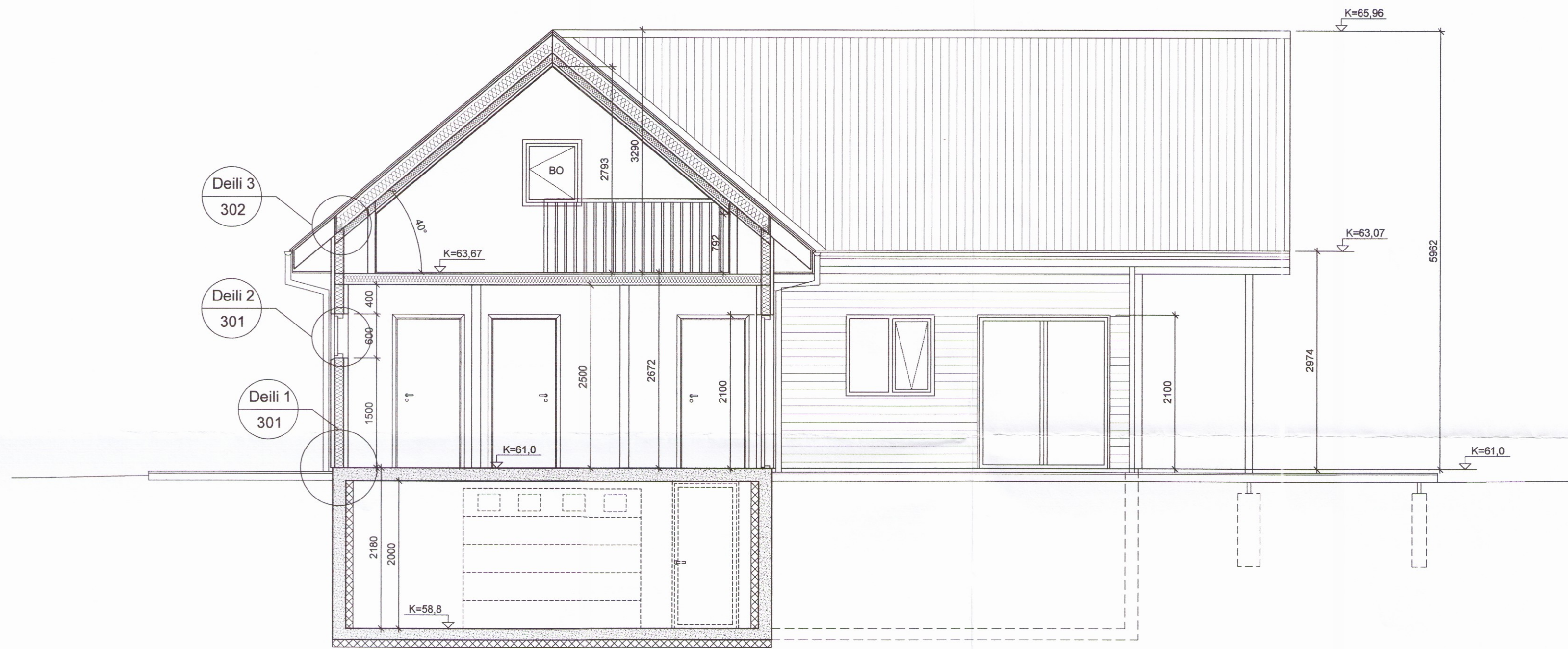
Sneiðing A-A 1:100
