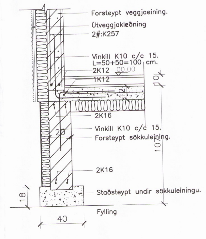
B Snið B-B. 1:20.
