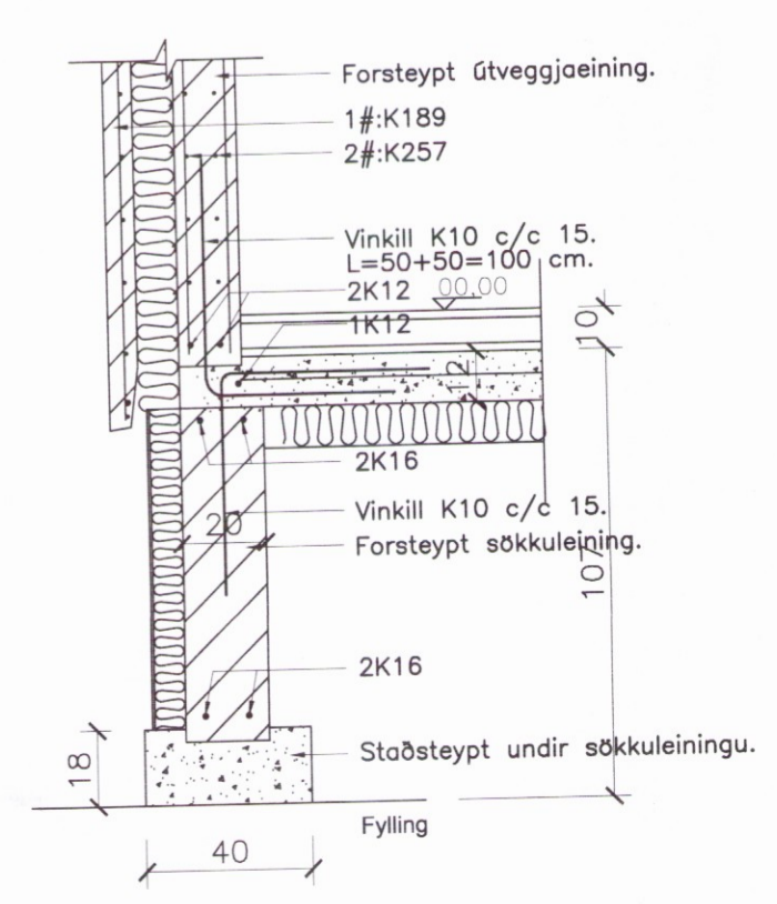
A Snið A-A. 1:20.
