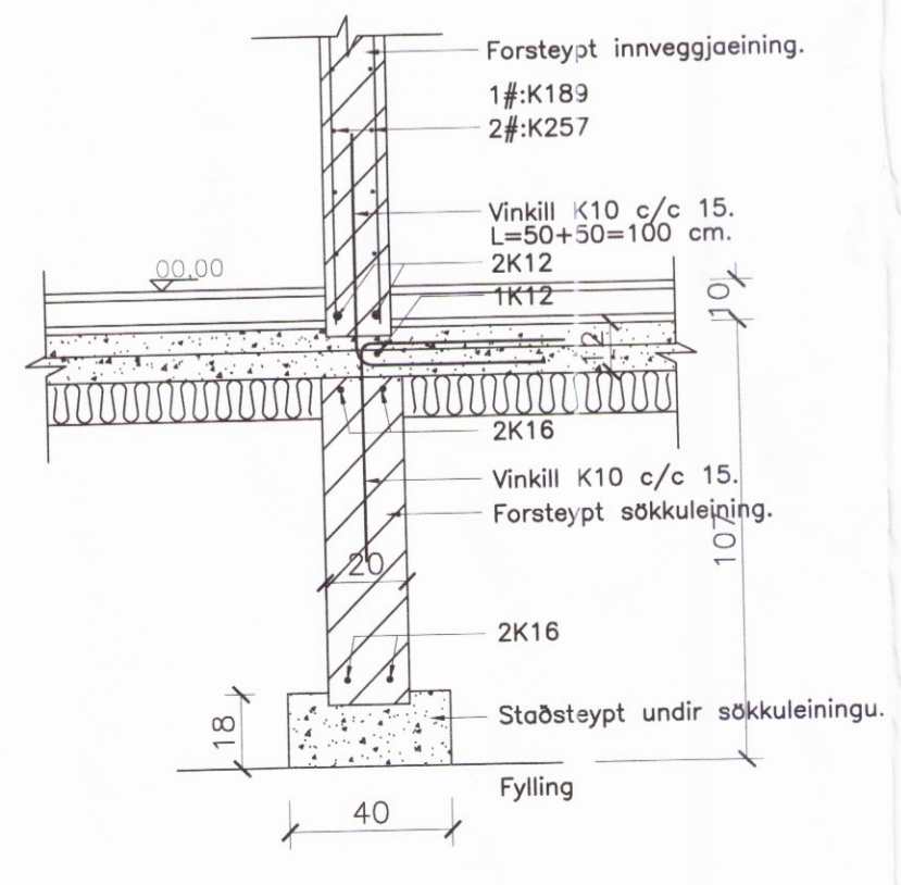
C Snið C-C. 1:20.
