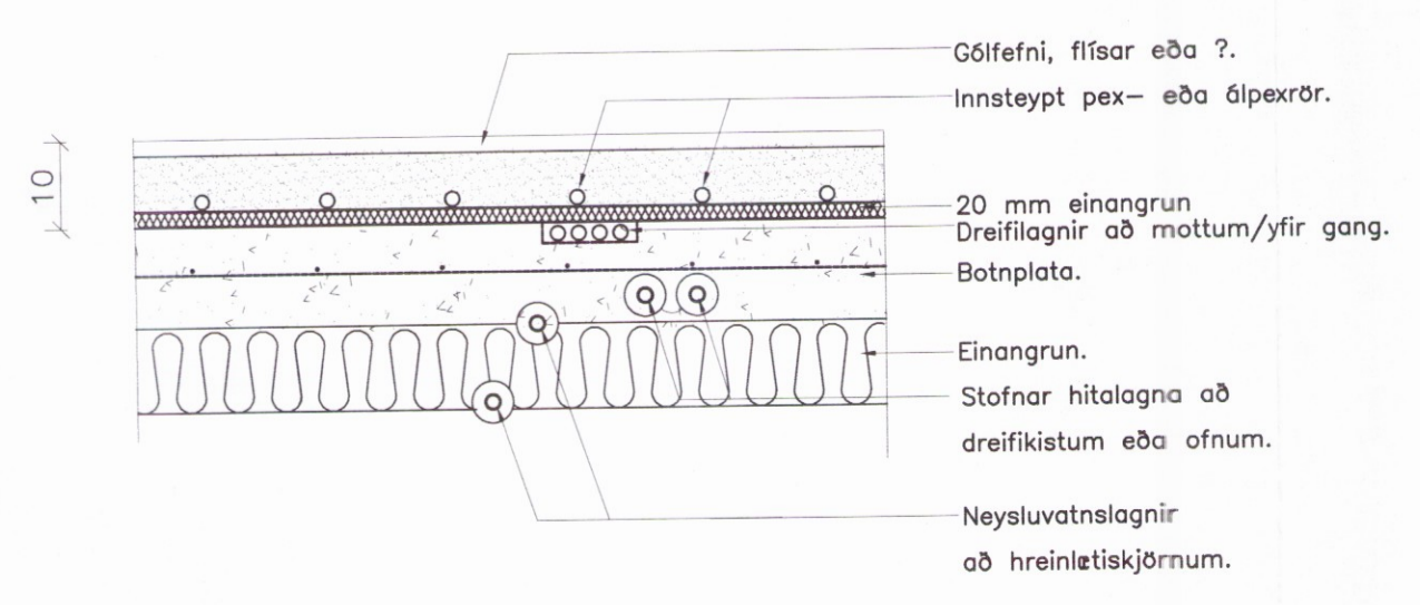
Snið í gólf. 1:10
