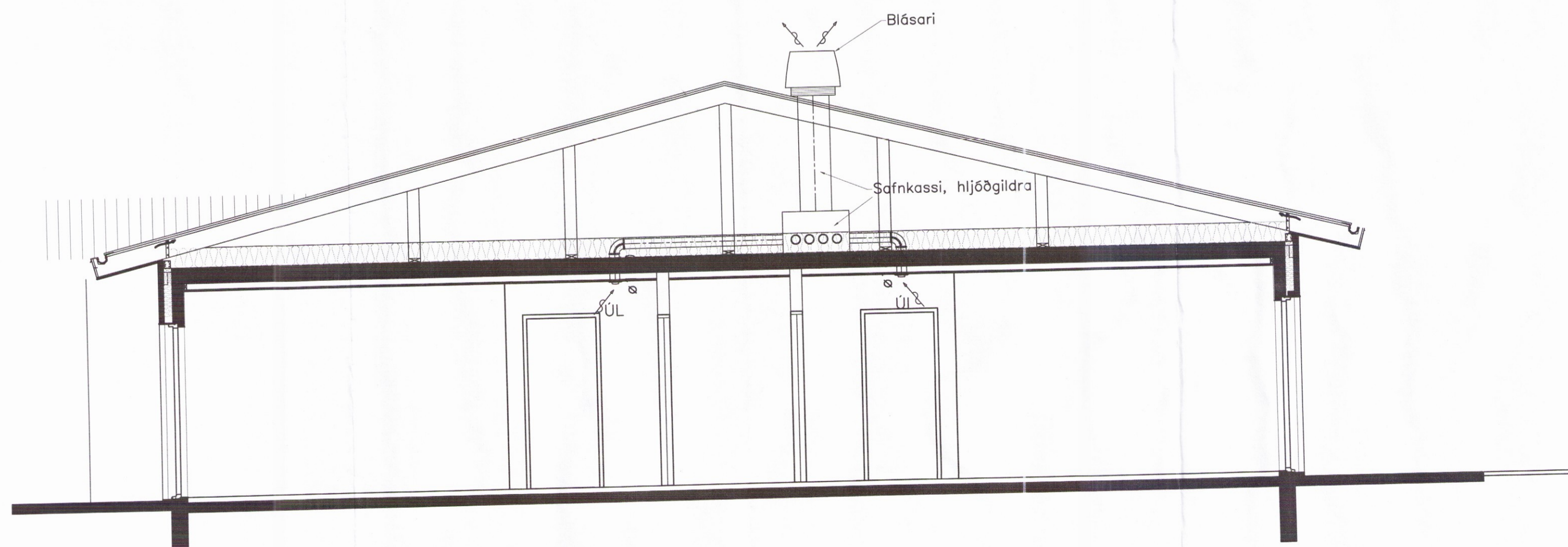
Sneiðing A-A 1:50
