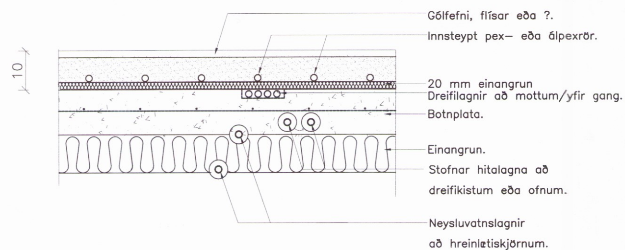
Snið 10-10 í gólf. 1:10
