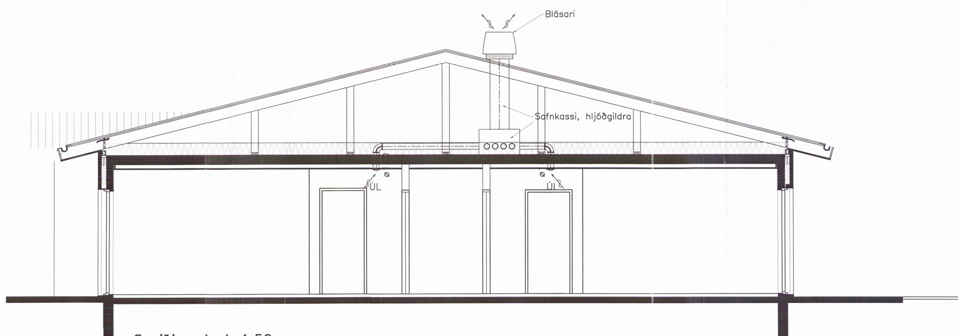
Sneiðing A-A 1:50
