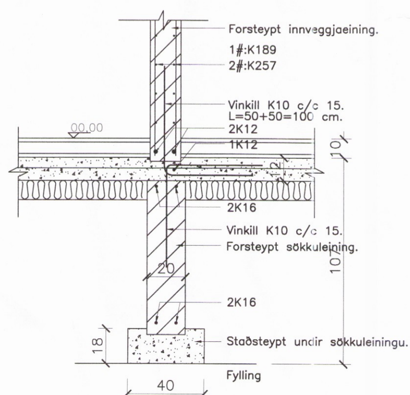
C Snið C-C. 1:20.
