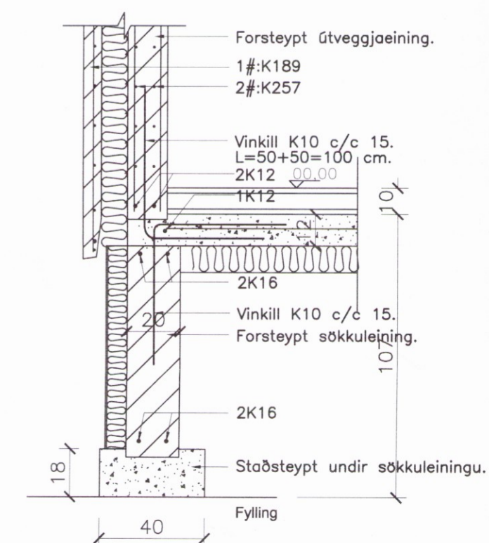
A Snið A-A. 1:20.
