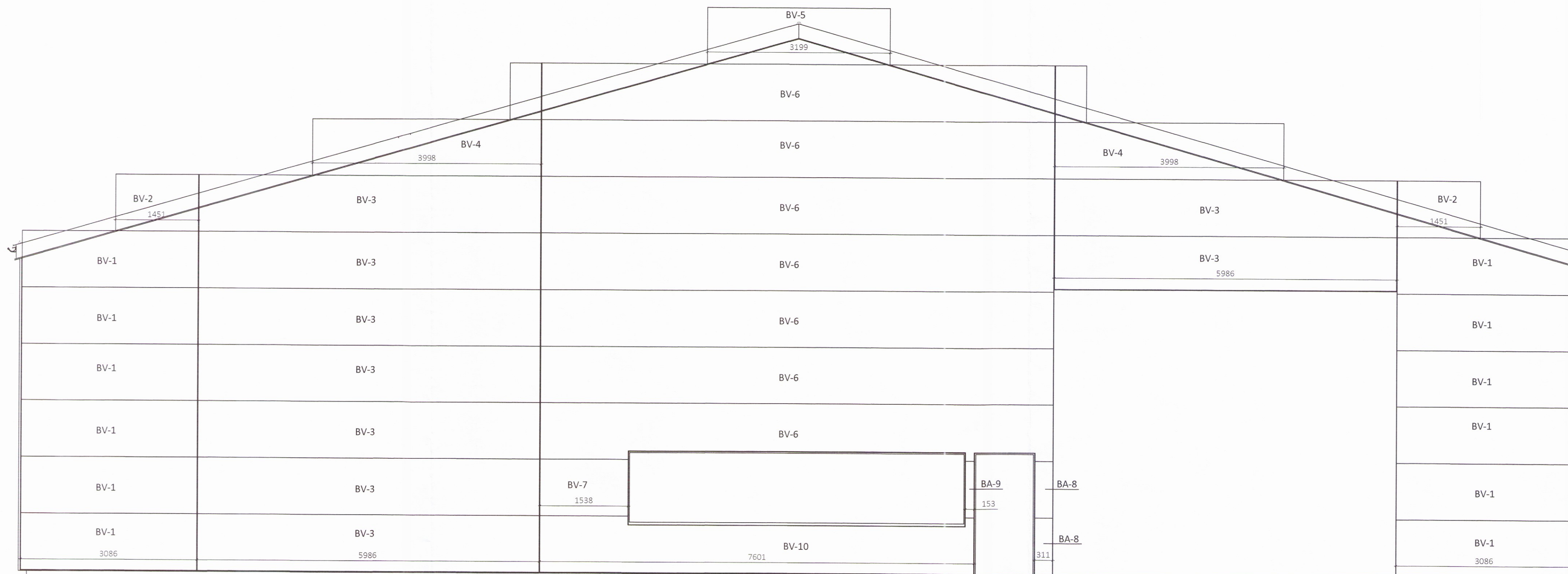
Vesturhlið Mkv. 1:50
