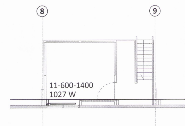
GRUNNMYND 2. HÆÐAR M1:100
